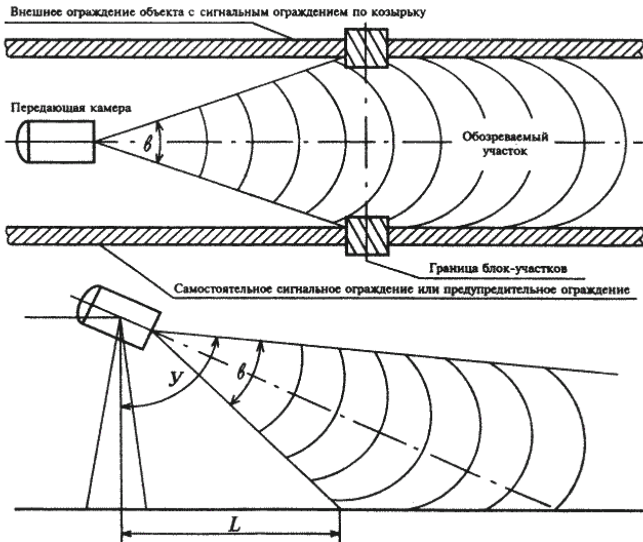
Рис. 1. Схема размещения камеры ПТУ
