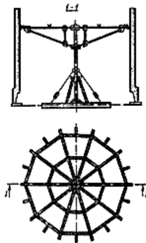
Рис.97. Кондуктор стационарного типа
