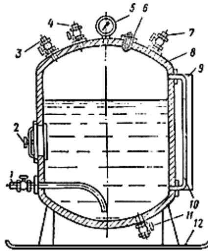
Рис.68. Схема пневматической установки для нагнетания закрепляющих растворов в грунты
