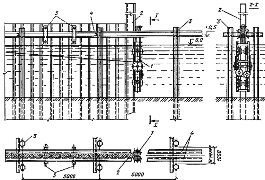
Погружение железобетонного шпунта с использованием прижимной тележки
