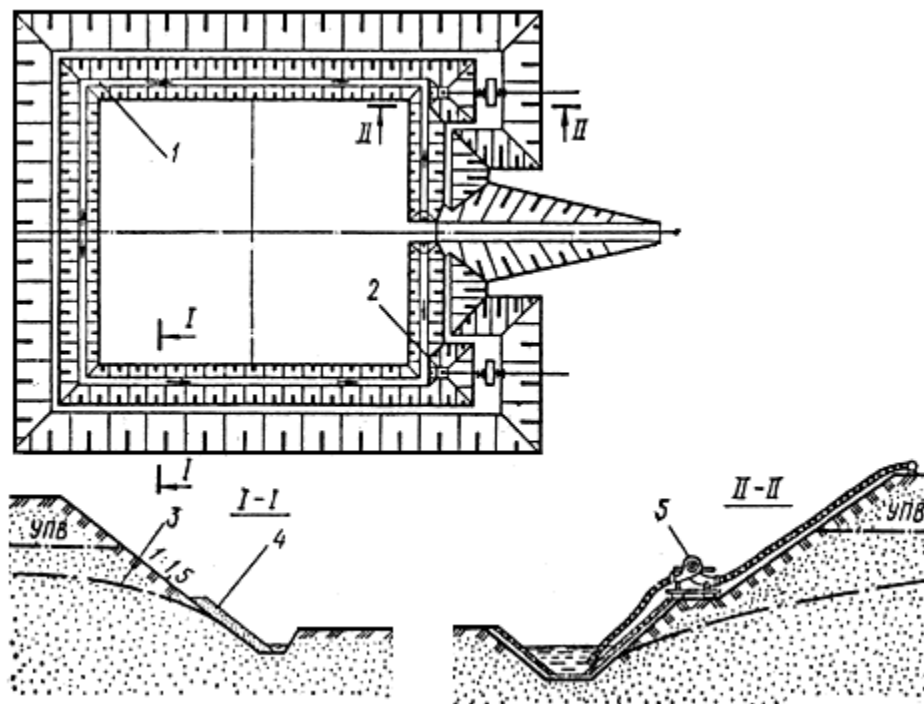
Рис.31. Открытый водоотлив в котловане
