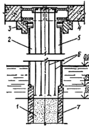
Рис.3. Свая-оболочка со стальным верхним звеном, бетонируемым "насухо" 1 - песок заполнения; 2 - бетон; 3 - сборная капитель; 4 - верхнее строение; 5 - стальная труба; 6 - армированный каркас; 7 - свая-оболочка
