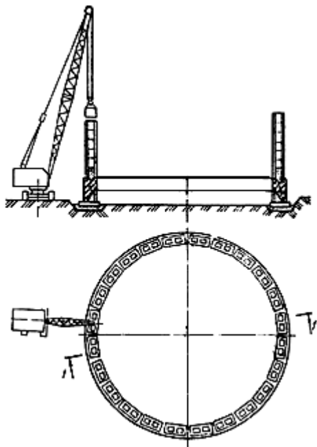
Рис.96. Монтаж сборно-монолитного колодца из пустотных блоков После окончания монтажа второго ряда блоков их пустоты следует заполнить бетоном марки М200 на высоту 400-500 мм.
