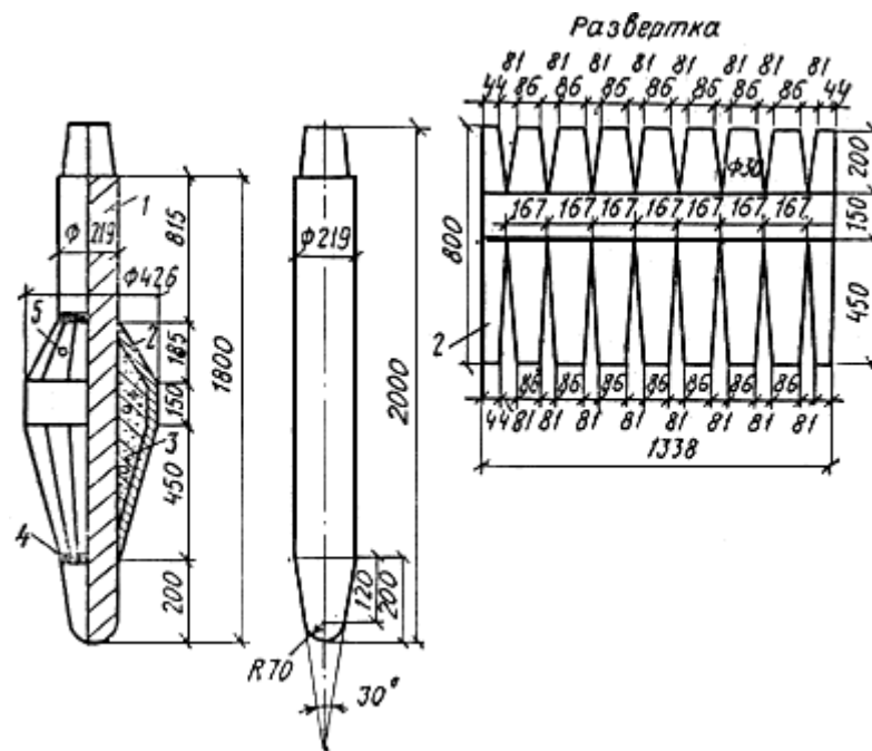
Рис.8. Конструктивная схема наконечника для пробивки скважин 1 - сердечник-долото; 2 - оболочка; 3 - бетон; 4 - сварные швы; 5 - отверстие для подачи бетонной смеси под оболочку
