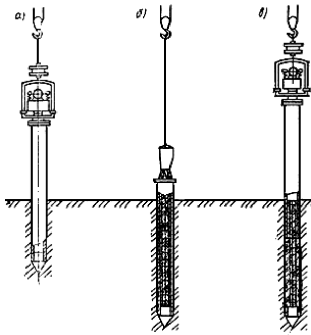
Рис.3. Изготовление набивных свай без выемки грунта
