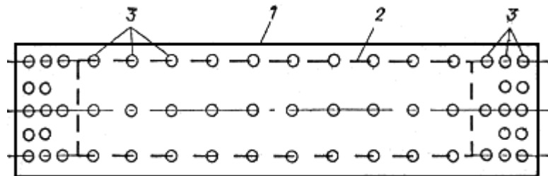
Рис.25. Рекомендуемая схема расположения скважин для замачивания котлованов
