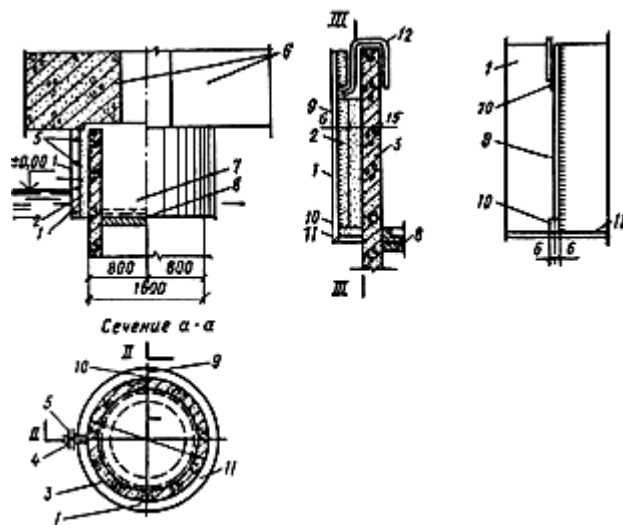
Рис.5. Теплогидроизоляционная защита из битумно-минеральной смеси (БМС) железобетонных свай-оболочек
