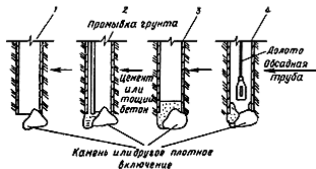
Рис.6. Рекомендуемые мероприятия по предупреждению искривлений скважин
