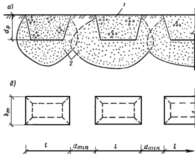
Рис.2. Ленточные прерывистые фундаменты в вытрамбованных котлованах
