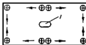
Рис.112. Схема бермы у консоли кессона при разработке грунта
