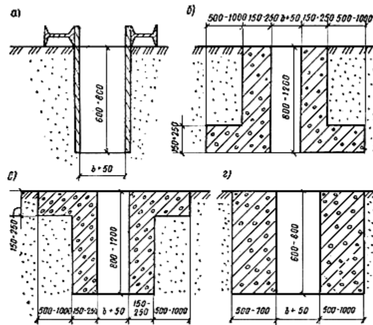
Рис.80. Конструкции крепления верха траншей
