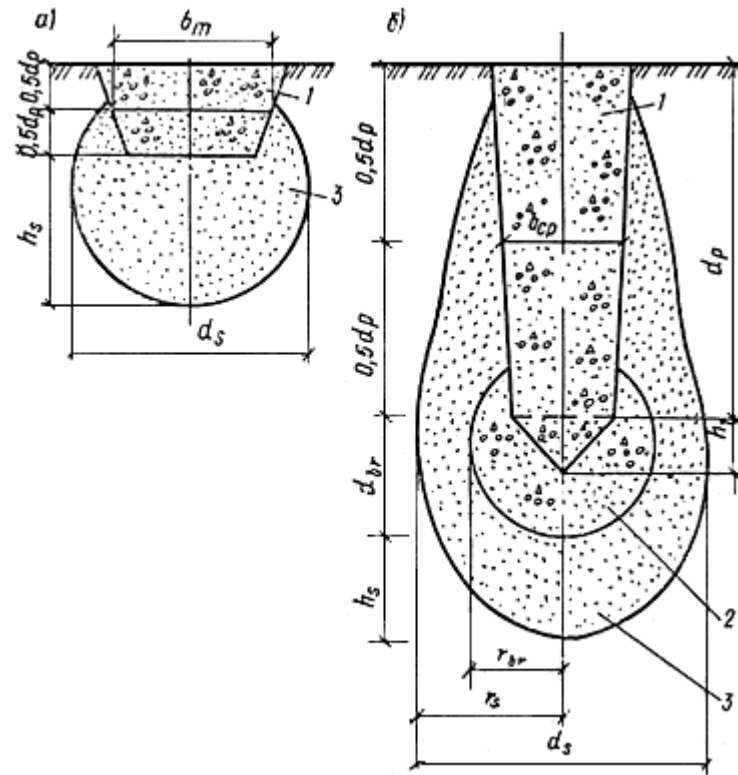
Рис.1. Фундаменты в вытрамбованных котлованах
