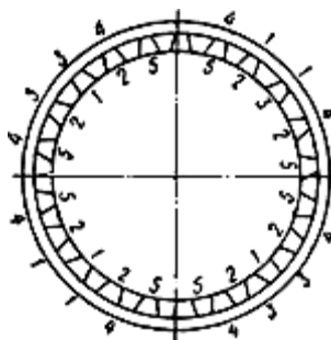
Рис.95. Последовательность снятия колодцев с опорного кольца
