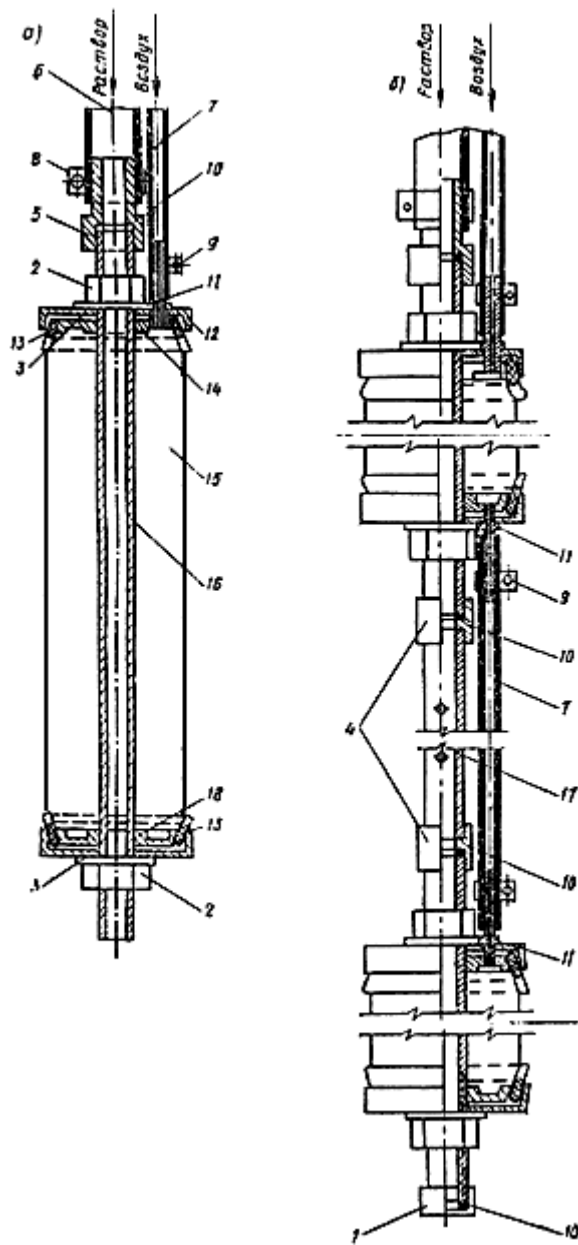
Рис.61. Инъекторы-тампоны пневматические
