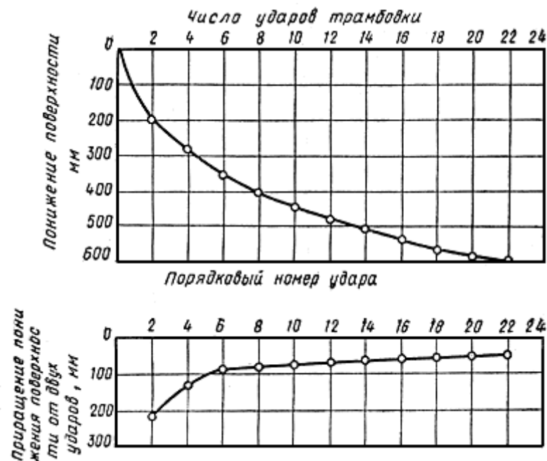
Рис.13. Графики понижения трамбуемой поверхности
