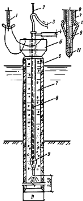
Рис.1. Схема вибропогружения свай-оболочки с применением пневмоинъектора 1 - крюк плавкрана; 2 - строп к крюку плавкрана; 3 - гибкий шланг к водяному насосу; 4 - гибкий шланг к воздушному компрессору; 5 - вибропогружатель; 6 - свая-оболочка; 7 - воздуховод; 8 - подмывная труба; 9 - соединительный наконечник с соплами; 10 - отверстия для выхода воздуха; 11 - сопла для воды
