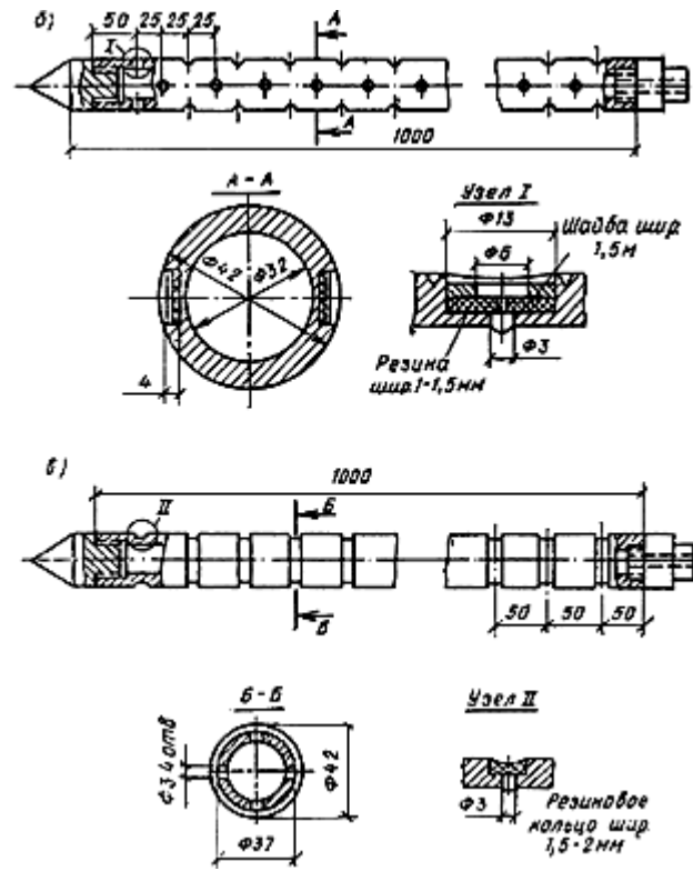
Рис.58. Конструкция забивного иньектора для силикатизации и смолизации песчаных грунтов
