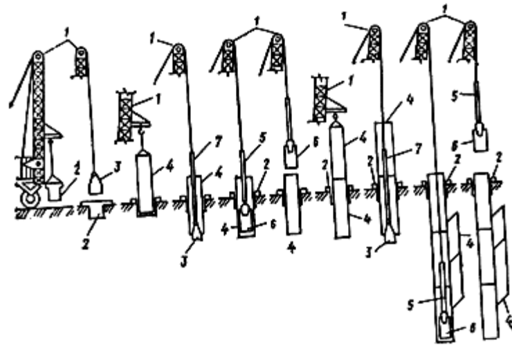
Рис.3. Устройство скважин станком ударно-канатного бурения 1 - буровая установка; 2 - кондуктор; 3 - долото;
