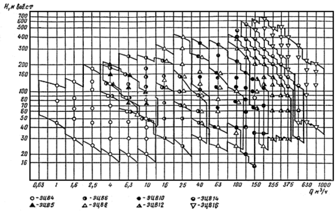
Рис.29. Характеристика насосов типа ЭЦВ
