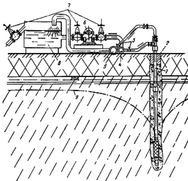
Рис.50. Установка ЭИ-70 с эжекторными иглофильтрами
