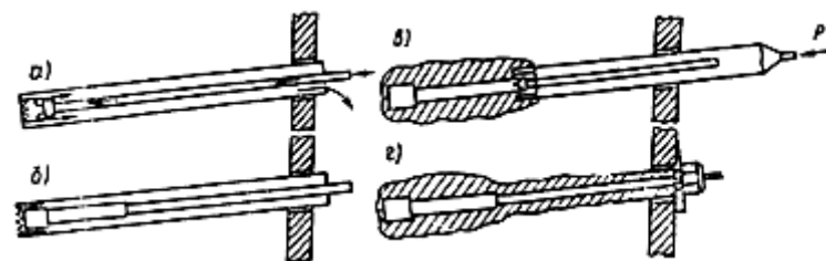
Рис.2. Технология устройства анкера с опорной трубой
