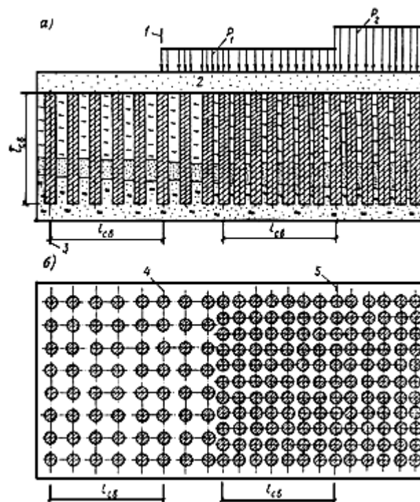
Рис.73. Относительное расположение границ зон действующих нагрузок и свайных полей с различной несущей способностью
