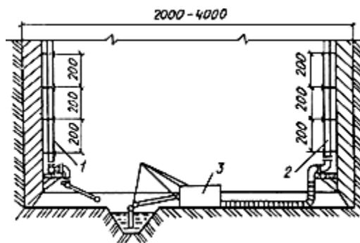
Рис.105. Разработка грунта землесосом
