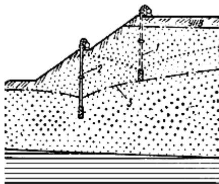
Рис.45. Схема ярусного водопонижения иглофильтрами
