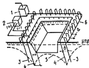
Рис.53. Схема электроосушения грунтов
