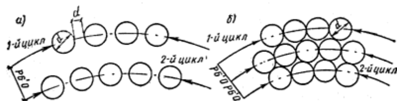
Рис.22. Схема уплотнения в пределах отдельного участка
