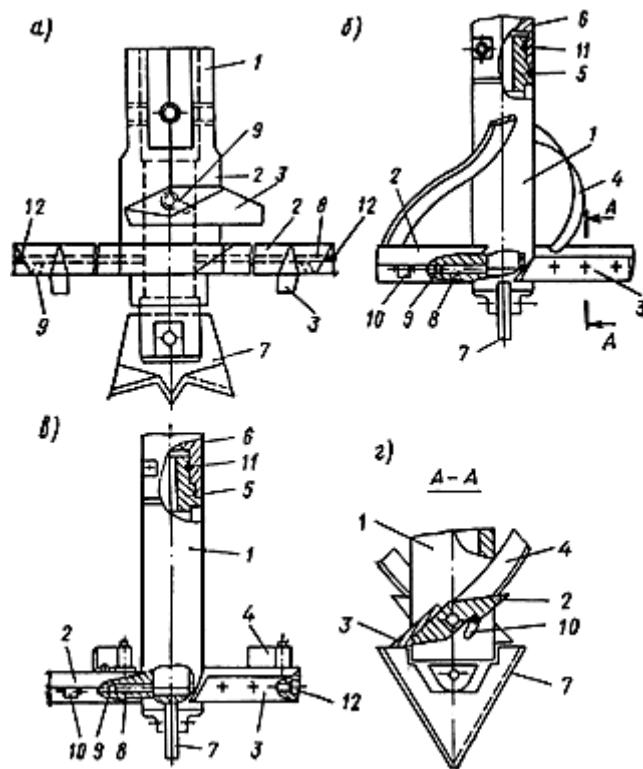
Рис.71. Схемы буросмесителей
