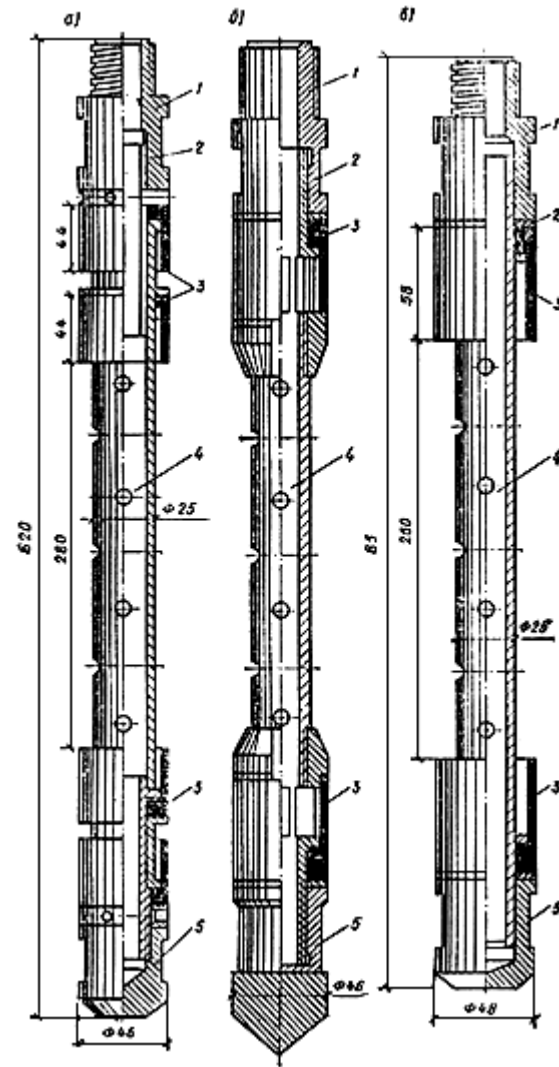
Рис.63. Конструкции манжетных тампонов
