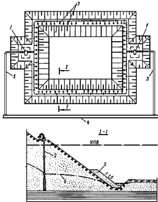
Рис.44. Контурная система иглофильтров
