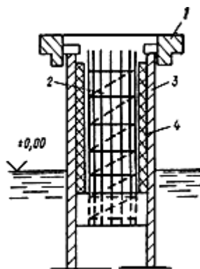
Рис.6. Схема устройства амортизирующего слоя на свае-оболочке
