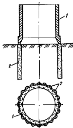
Рис.90. Устройство песчаных свай под ножом по периметру колодца в слабых грунтах 1 - опускной колодец; 2 - песчаные сваи
