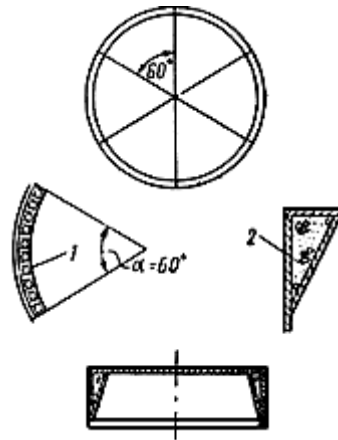
Рис.108. Ножевая часть опускного колодца
