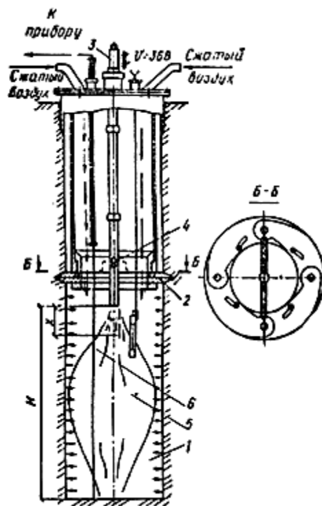
Рис.74. Схема термического закрепления грунтов с применением многоспайной термопары и винтообразного отсекателя рабочего объема скважины 1 - нагревательная скважина; 2 - отсекающий; 3 - форсунка; 4 - удлинитель форсунки; 5 - факел горения смесей; 6 - термопары; 7 - запальник
