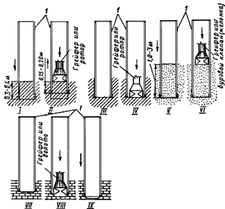
Рис.7. Рекомендуемые схемы взаимного расположения забоя и режущего наконечника 1 - обсадная труба
