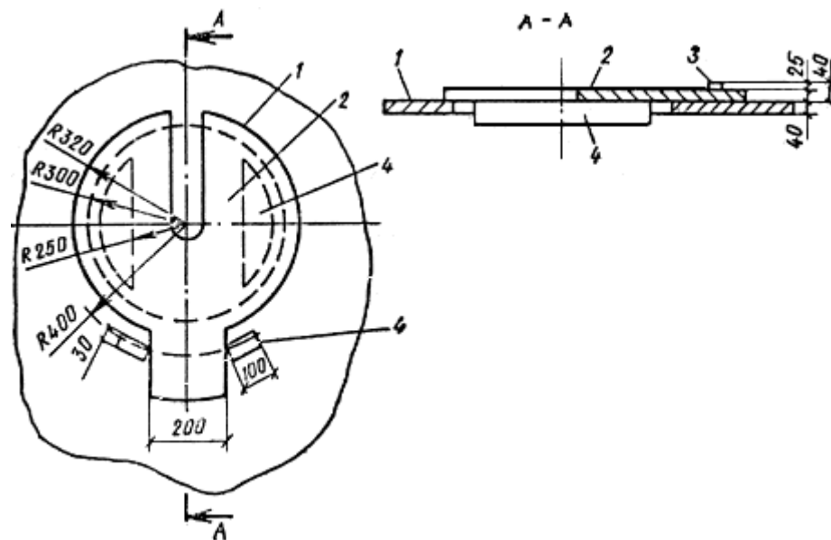
Рис.9. Новая поворотная плита для свинчивания штанг ударного снаряда
