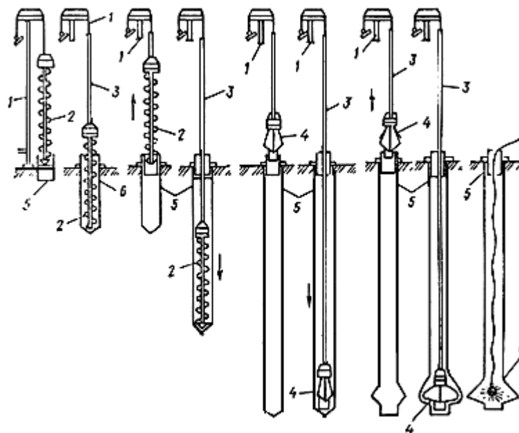
Рис.2. Разбуривание уширения скважины 1 - буровой станок; 2 - шнек; 3 - штанги; 4 - буровой уширитель; 5 - обсадной кондуктор; 6 - электролампа для осмотра скважины
