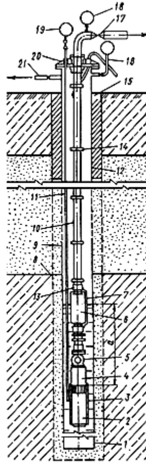
Рис.40. Вакуум-скважина
