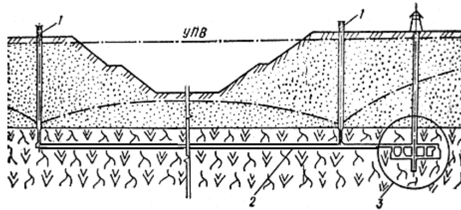
Рис.39. Система водопонижения со сквозными фильтрами
