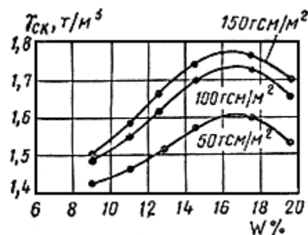
Рис.14. Графики зависимости удельного веса сухого грунта от влажности при постоянной удельной работе A ( A = 50, 100, 150 т·см/м)
