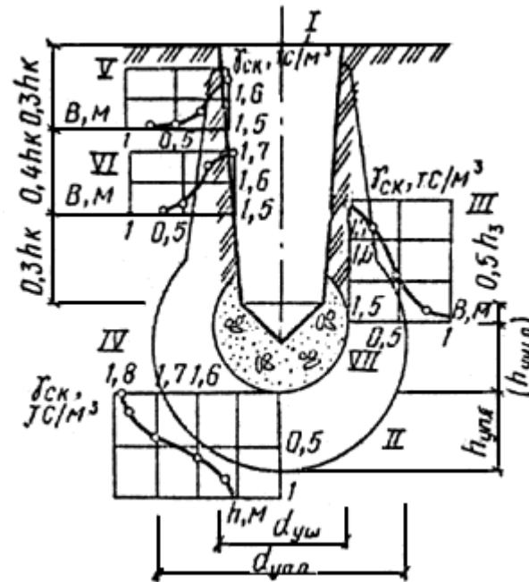
Рис.17. Уплотненная зона и график изменения объемного веса скелета уплотненных грунтов для удлиненных фундаментов с уширенным основанием I - вытрамбованный котлован; II - уплотненная зона; III - по горизонтали от оси котлована или от уширения; IV - по вертикали ниже дна котлована или от уширения; V, VI - по горизонтали от боковой поверхности; VII - уширенное основание
