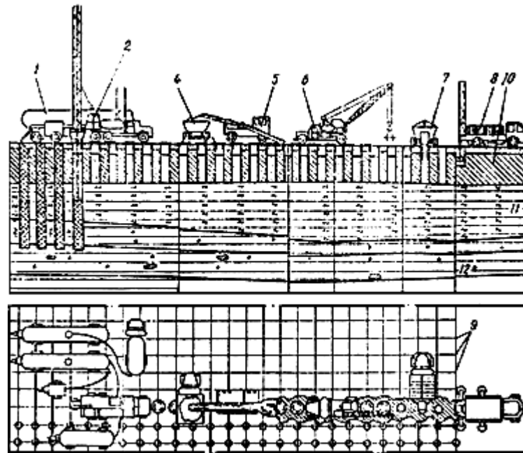
Рис.2. Укрепление основания бурсмесительным способом с использованием серийной буровой установки с передвижным растворонасосным узлом, с центральной буровой установки с передвижным растворонасосным узлом, снабжаемым цементным раствором с центрального бетонорастворного узла 1 - авторастворовоз типа СБ-89; 2 - передвижной растворонасосный узел; 3 - буровая установка типа УГБ-1ВС; 4 - автосамосвал ЗИЛ ММЗ-555; 5 - фронтальный погрузчик; 6 - автомобильный кран типа КС-2561Е; 7 - спецмашина; 8 - буровая установка; 9 - разбивочная сетка для илоцементных свай; 10 - перекрывающий слой; 11 - ил; 12 - твердые глины
