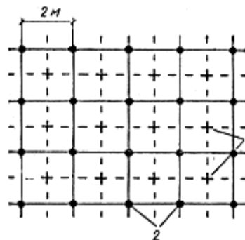
Рис.26. Схема расположения точек рыхления и уплотнения
