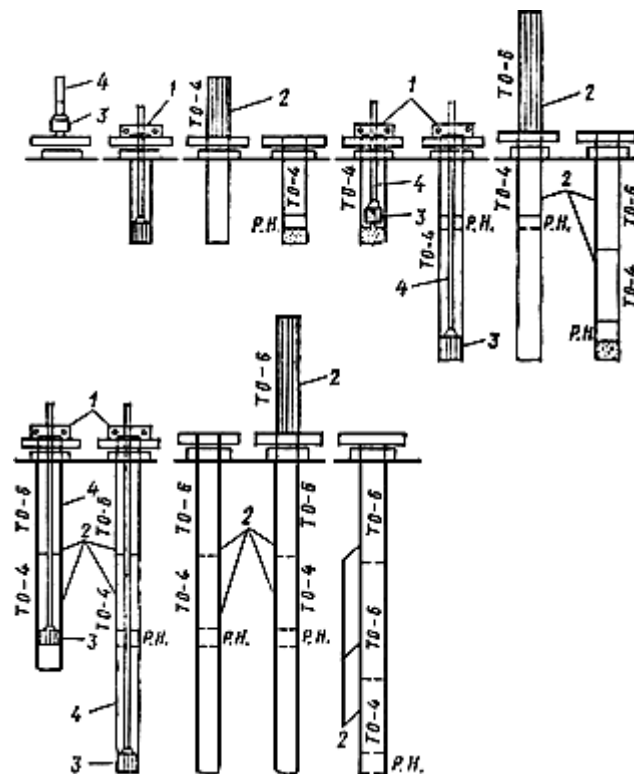
Рис.5. Устройство скважин буровыми станками типа СП-45
