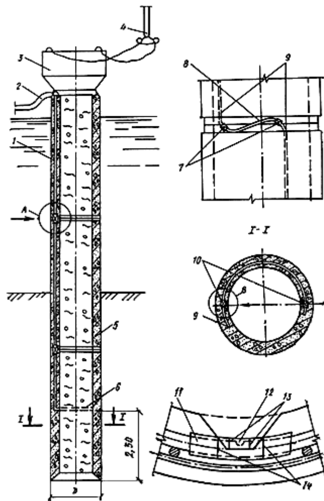
Рис.2. Схема вибропогружения сваи-оболочки с устройством воздухоподачи 1 - воздухопроводящая трубка; 2 - гибкий шланг к компрессору; 3 - вибропогружатель;
