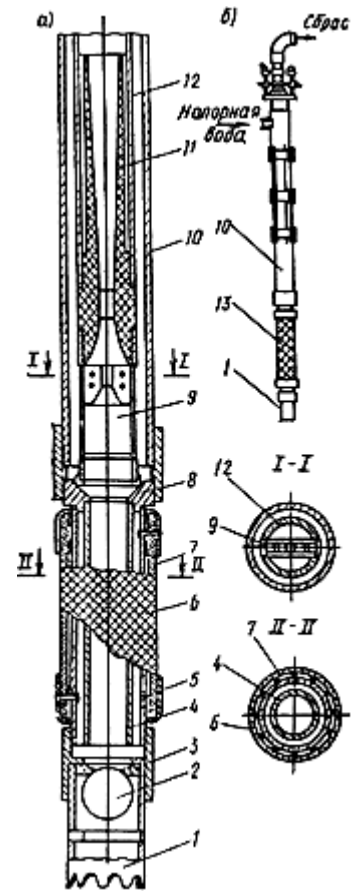
Рис.51. Эжекторный иглофильтр
