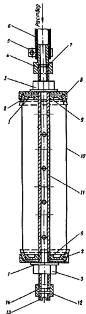
Рис.60. Инъектор-тампон гидравлический, одинарный для силикатизации просадочных лессовых грунтов в скважинах
