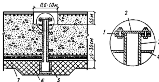
Рис.106. Устройство для откачки грунтовых вод из-под дна
