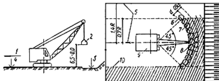
Технологическая карта производства работ по поверхностному уплотнению грунтов 1 - направления движения крана; 2 - железобетонная трамбовка; 3 - проектная отметка; 4 - отметка дна котлована перед трамбовкой; 5 - направление рабочего хода и ось движения крана; 6 - первый цикл (два удара); 7 - второй цикл (два удара); 8 - полоса, уплотняемая с одной стоянки крана; 9 - стоянка крана через 0,9d ; 10 - уплотненный грунт
