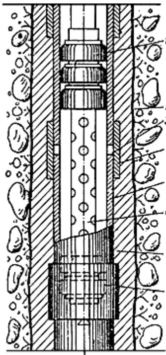
Рис.62. Схема манжетно-тампонного иньектора 1 - манжетный тампон с перфорированной частью 6; 2 - стенка скважины; 5 - колонна труб с отверстиями 3 и резиновыми кольцами 4; 7 - обойменный глиноцементный раствор
