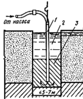
Рис.87. Схема заполнения секции траншеи глиноцементным раствором 1 - труба диаметром 50 мм; 2 - глинистая суспензия; 3 - глиноцементный раствор
