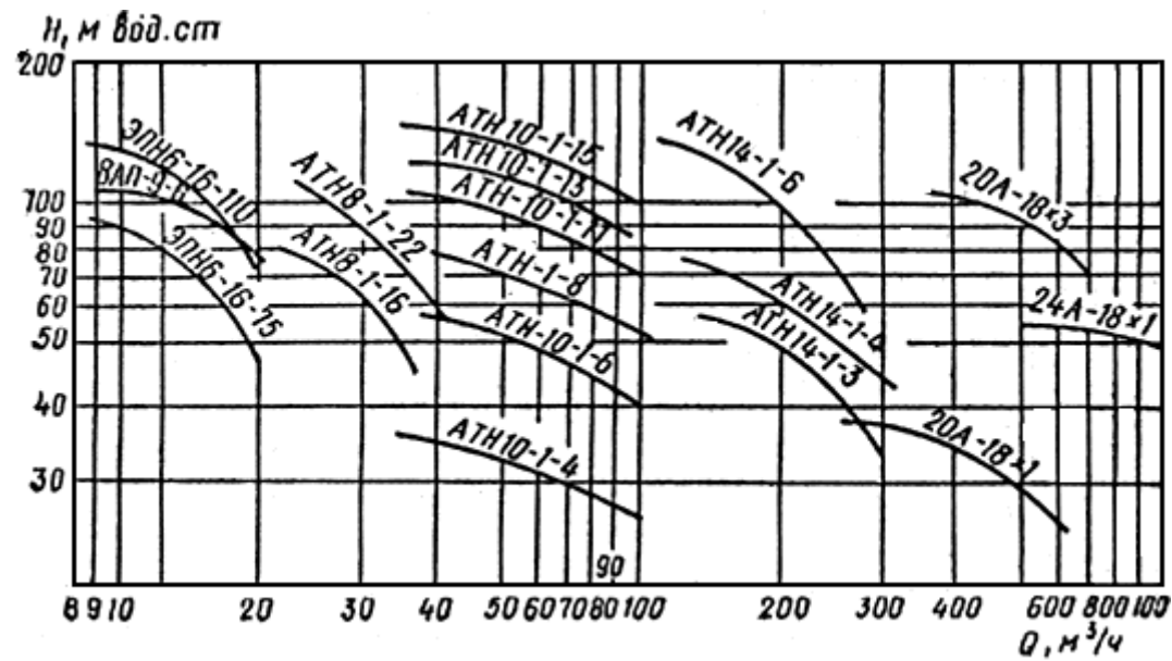
Рис.30. Характеристики насосов типа А, АП, АТН, ЭПН
