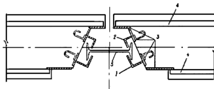
Рис.84. Съемная (инвентарная) направляющая
