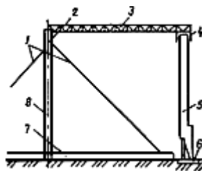
Рис.98. Кондуктор консольного типа
