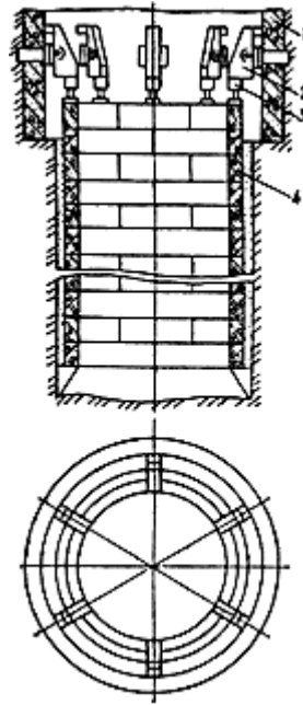
Рис.110. Задавливание колодца посредством угловых упоров
