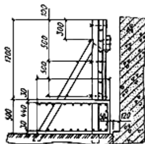
Рис.100. Конструкция ограждения форшахты
