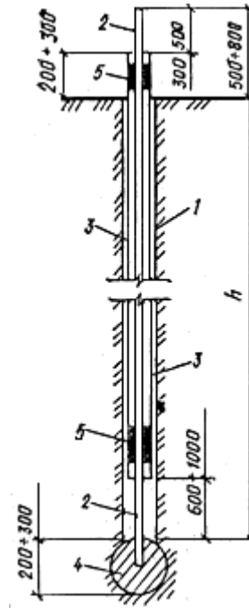
Рис.20. Конструкция глубинной марки
