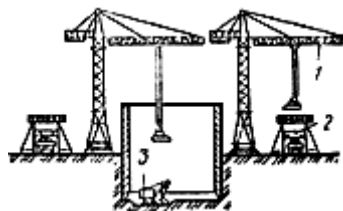
Рис.104. Разработка грунта экскаватором 1 - башенный кран; 2 - бункер; 3 - экскаватор
