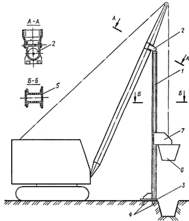
Рис.3. Схема оборудования для вытрамбовывания котлованов на экскаваторе со стрелой драглайн 1 - направляющая штанга; 2 - шарнир; 3 - упорная плита; 4 - зубья; 5 - направляющая пластина; 6 - трамбовка; 7 - каретка
