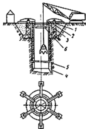
Рис.107. Технологическая схема погружения колодца способом задавливания
