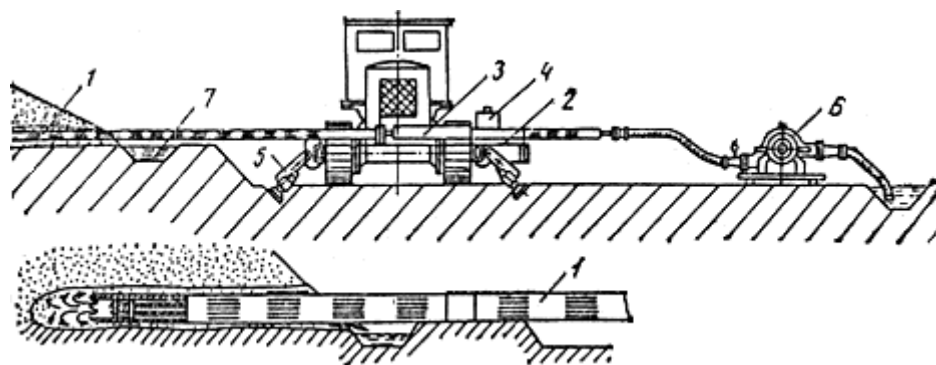
Рис.35. Схема устройства горизонтальной скважины
