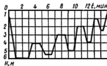
Рис.27. Технологический график уплотнения песчаного грунта
