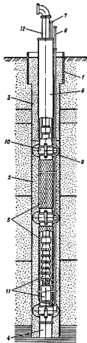
Рис.33. Открытая скважина, оборудованная насосом
