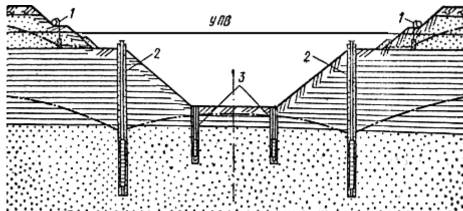
Рис.34. Система водопонижения с применением резервных самоизливающихся скважин
