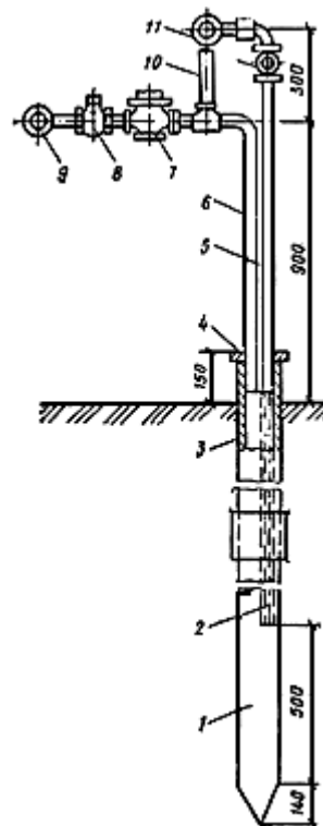
Рис.78. Замораживающая колонка
