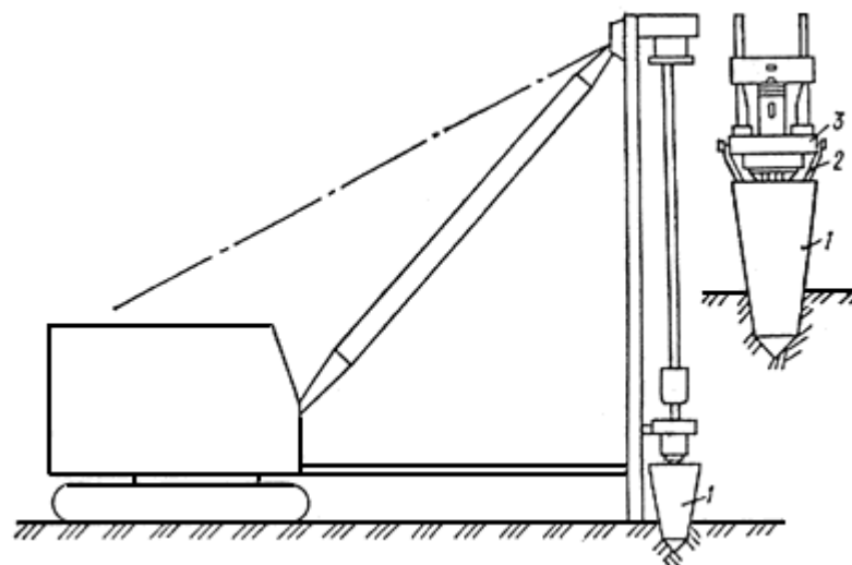
Рис.7. Схема оборудования для вытрамбовывания котлованов на базе сваебойного агрегата
