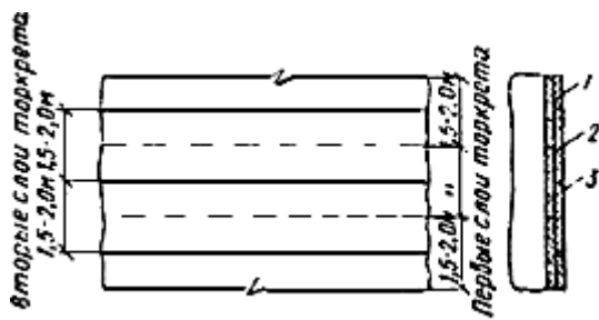
Рис.92. Порядок нанесения слоев торкрет-гидроизоляции 1 - 1-й слой торкрета; 2 - 2-й слой торкрета; 3 - битумный слой
