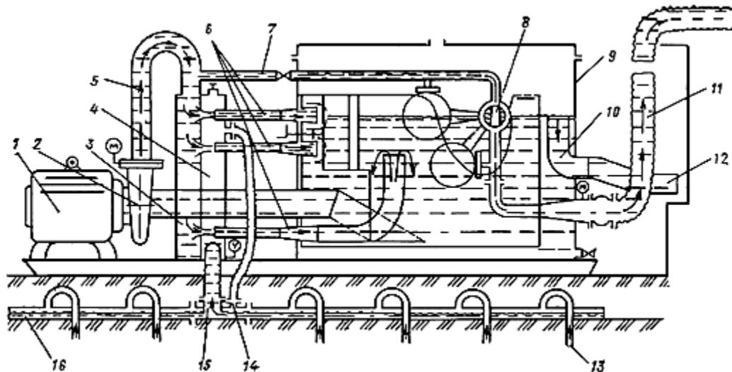
Рис.49. Схема насосной установки УВВ-3
