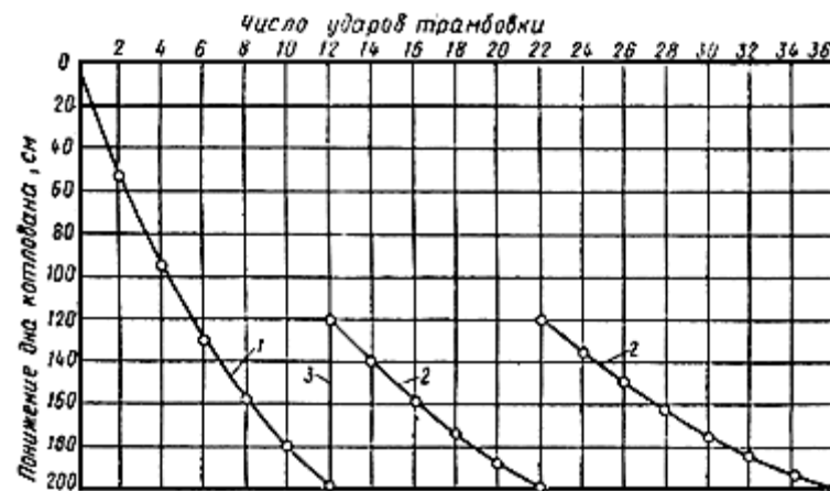
Рис.15. Понижение дна котлована в процессе вытрамбовывания и втрамбовывания жесткого материала 1 - вытрамбовывание; 2 - втрамбовывание жесткого материала; 3 - засыпка жесткого материала
