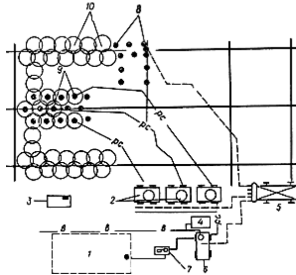
Рис.56. Схема организации работ по закреплению грунтов через инъекторы 1 - место складирования химреагентов; 2 - пневмоустановки (или насосы); 3 - верстак; 4 - емкость с водой; 5 - компрессор; 6 - емкость для приготовления рабочих растворов; 7 - насос; 8 - погруженные инъекторы; 9 - нагнетание закрепляющих растворов; 10 - закрепленный грунт; В - вода; РС - закрепляющие растворы или смеси
