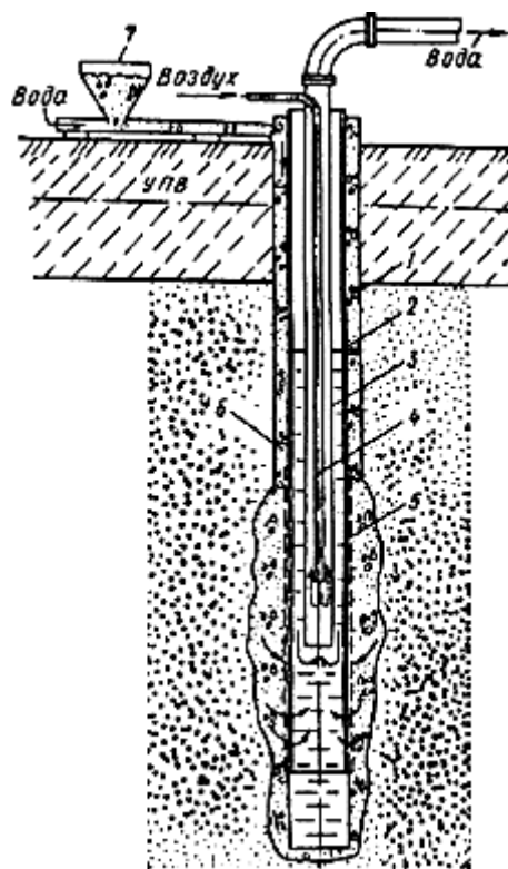
Рис.42. Схема устройства гидравлическим способом песчано-гравийной обсыпки скважины 1 - обсадные трубы; 2 - надфильтровые трубы; 3 - водоподъемные трубы; 4 - воздушная труба; 5 - фильтр; 6 - песчано-гравийная обсыпка; 7 - бункер для обсыпки
