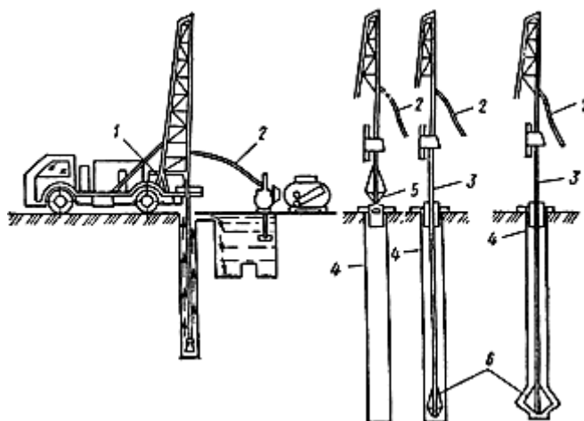
Рис.4. Устройство скважины буровым станком под глинистым раствором 1 - буровой станок типа УРБ-ЗАМ; 2 - шланг, подающий глинистый раствор; 3 - буровые штанги; 4 - направляющий кондуктор; 5 - шарошечное долото; 6 - буровой ушитель (для скважин с глинистым раствором)
