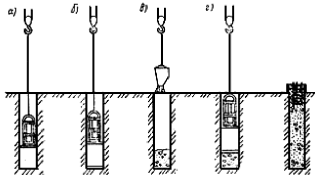
Рис.1. Изготовление набивных свай с помощью виброгрейферов
