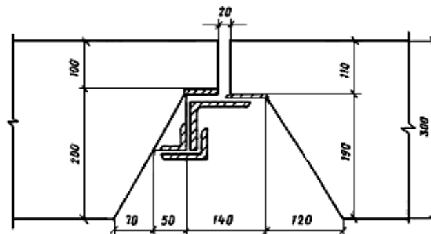
Рис.86. Стационарная направляющая
