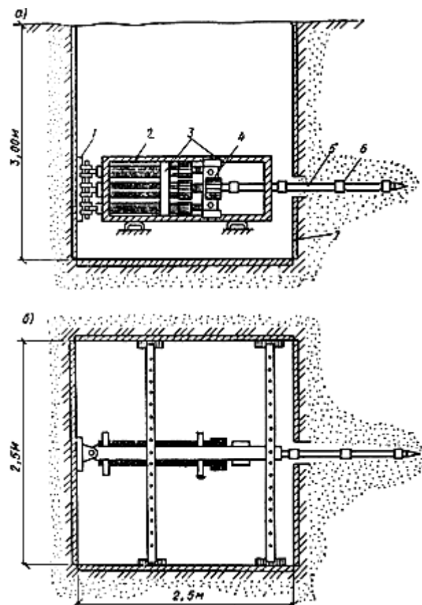
Рис.64. Схема гидравлического задавливания манжетно-тампонных иньекторов из технологических выработок при силикатизации и смолизации грунтов по горизонтальной технологии
