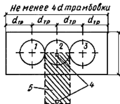
Рис.12. Схема размещения штырей для определения величины отказа
