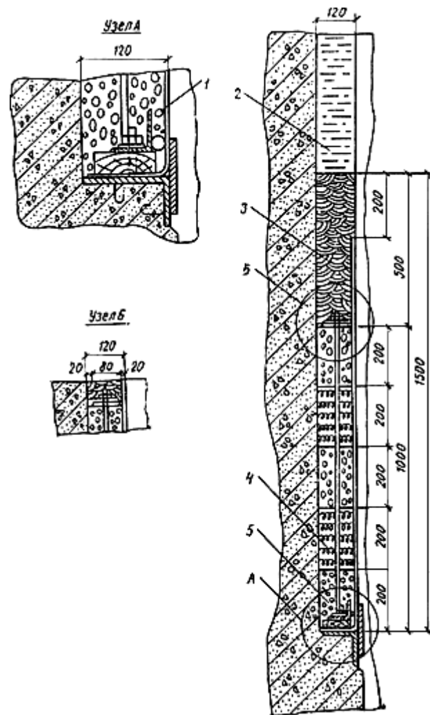
Рис.101. Пример конструкции замкового уплотнителя 1 - резинт;
