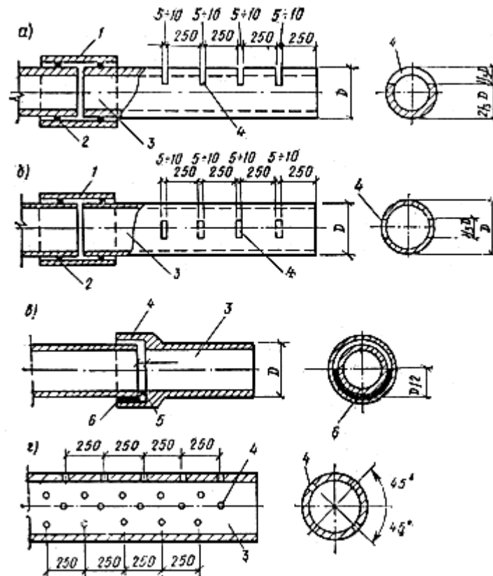
Рис.28. Водоприемные отверстия в дренажных трубах
