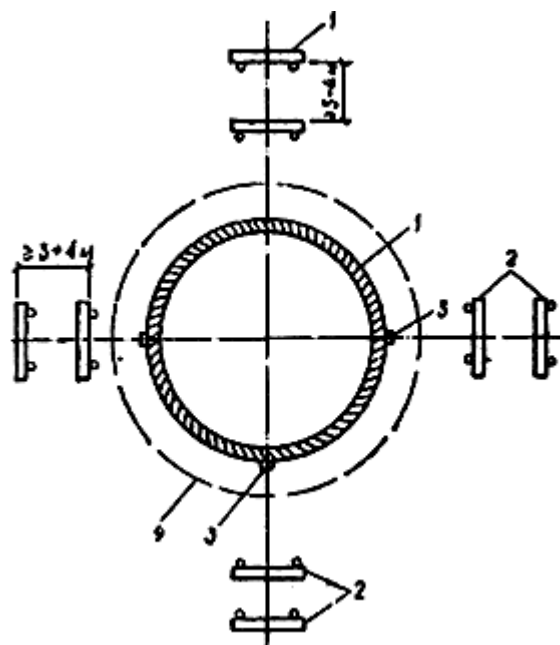
Рис.89. Схема закрепления основных осей опускного колодца или кессона на местности
