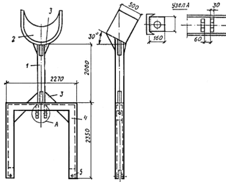
Рис.10. Дозатор (совок) емкостью 0,35 \text{ м}^3 для засыпки скважин грунтом
