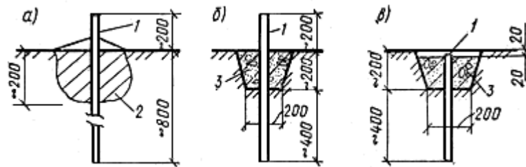
Рис.19. Конструкции поверхностных марок
