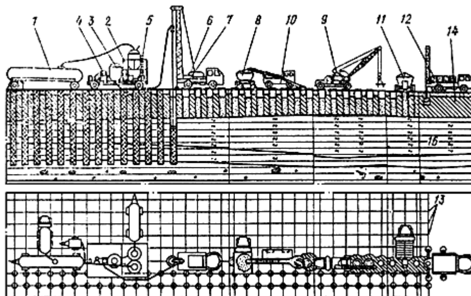
Рис.3. Укрепление основания буросмесительным способом с использованием серийной установки, с передвижным растворонасосным узлом, снабжаемым готовым цементным раствором с центрального бетонорастворного узла
