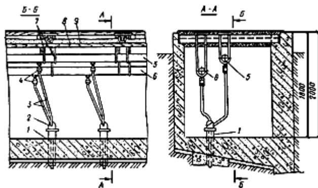
Рис.77. Расположение рассольных коммуникаций в форшахте
