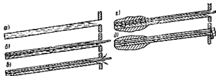
Рис.3. Технология устройства анкера с инъекционной трубкой
