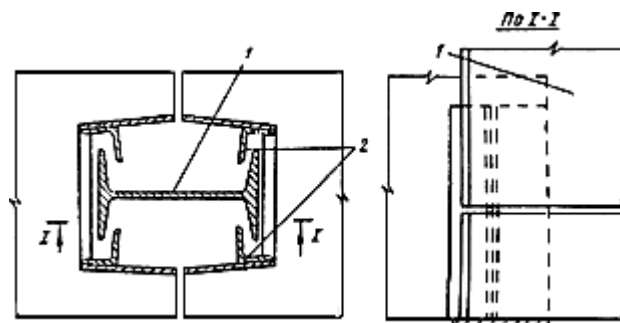
Рис.85. Стык панелей с прямоугольной разделкой шва
