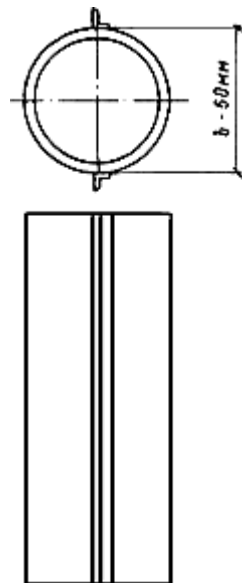
Рис.81. Трубчатый ограничитель
