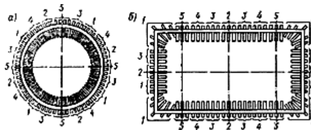
Рис.94. Последовательность снятия колодцев с деревянных подкладок
