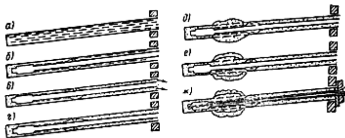
Рис.4. Технология устройства анкера с манжетной трубой при внутреннем расположении тяги с двухкратной инъекцией
