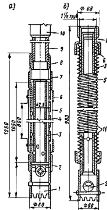
Рис.48. Конструкция иглофильтров
