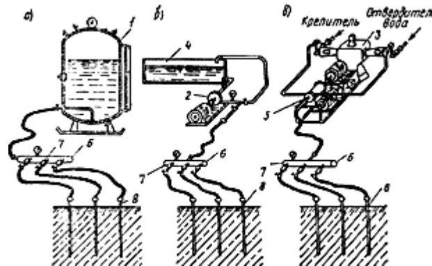
Рис.67. Технологические схемы нагнетания закрепляющих растворов в грунты
