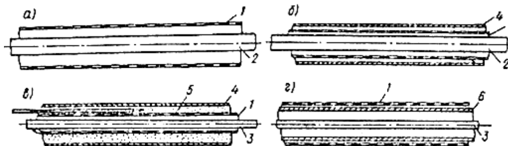
Рис.41. Схемы устройства горизонтальных скважин
