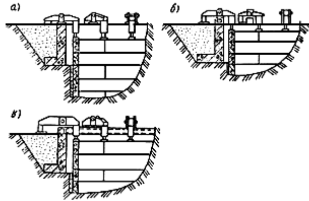
Рис.109. Устройство для задавливания опускного колодца
