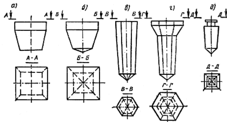
Рис.5. Основные виды трамбовок для вытрамбовывания котлованов
