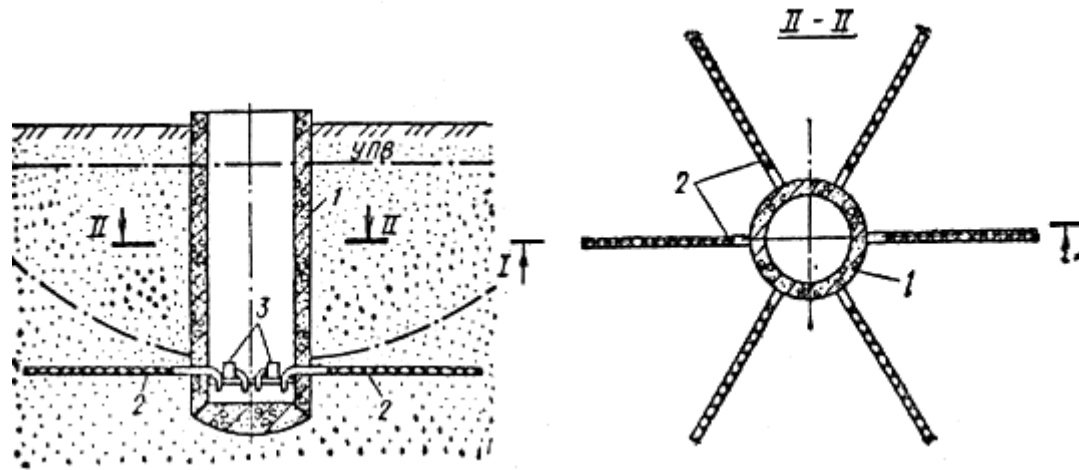
Рис.36. Лучевой водозабор
