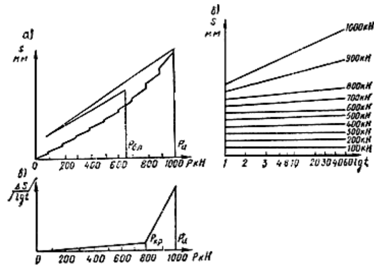
Рис.1. Контрольные испытания анкеров
