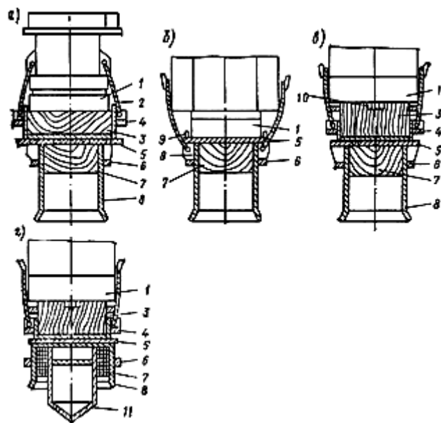
Схемы наголовников
