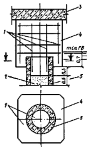
Рис.4. Свая-оболочка с монолитной железобетонной капителью 1 - армированный каркас; 2 - песок заполнения; 3 - верхнее строение; 4 - монолитная капитель; 5 - свая-оболочка
