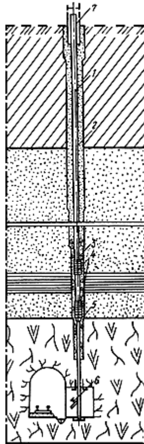
Рис.38. Сквозной фильтр
