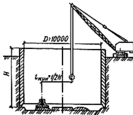
Рис.103. Схема разработки грунта в колодцах с использованием бульдозера и грейфера H - высота колодца
