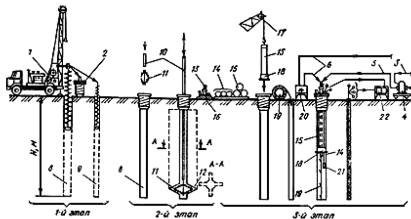
Рис.2. Технологическая схема выполнения основных этапов 1-3
