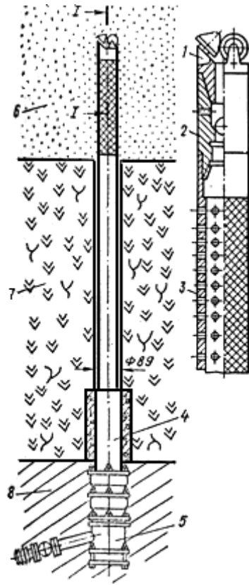
Рис.37. Восстающая скважина
