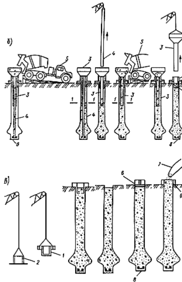
Рис.8. Бетонирование скважин для свай методом ВПТ
