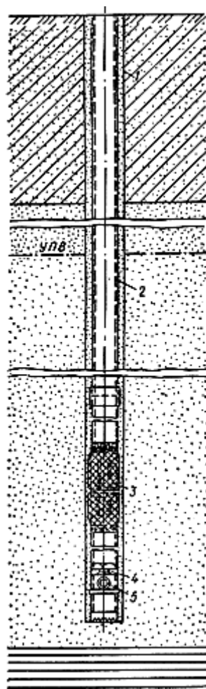
Рис.54. Наблюдательная скважина
