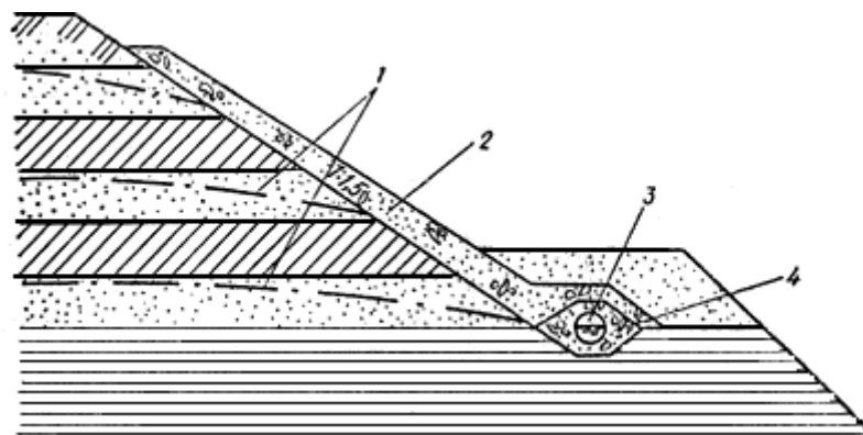
Рис.32. Дренаж на откосах котлована
