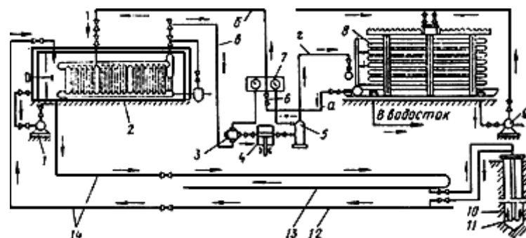
Рис.76. Схема работы замораживающей станции
