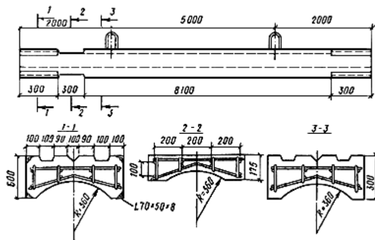
Рис.82. Незвлекаемый железобетонный ограничитель
