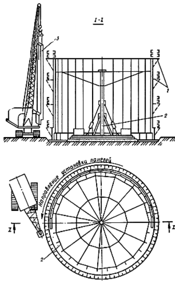
Рис.99. Монтаж сборного колодца из панелей 1 - подмости; 2 - кондуктор; 3 - сборная панель
