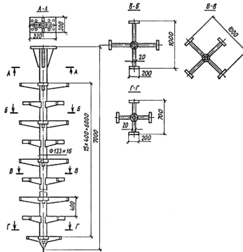
Рис.11. Уплотнитель виброустановки ВУУП-6
