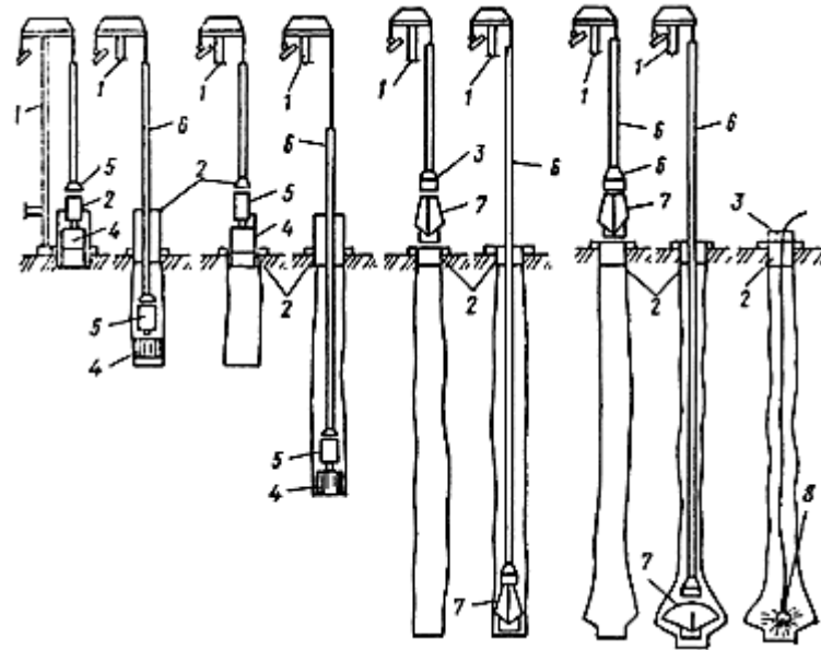
Рис.1. Бурение скважины шнеком
