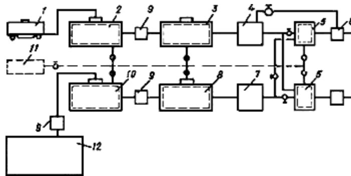
Рис.66. Технологическая схема приготовления гелеобразующей смеси при односторонней силикатизации и смолизации грунтов
