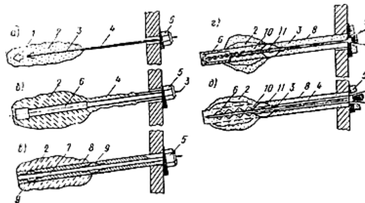
Принципиальные схемы анкеров
