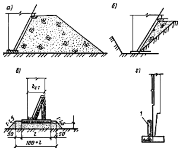
Рис.91. Конструкции временного основания под нож колодца
