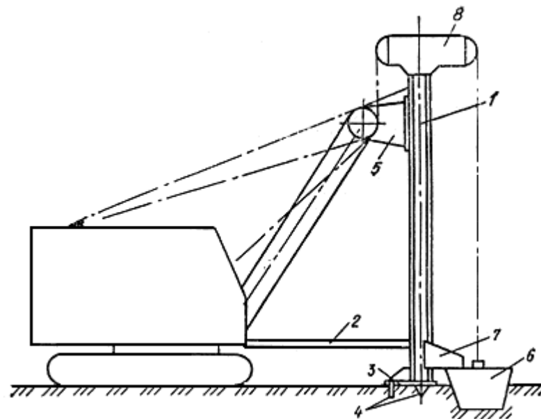
Рис.4. Схема оборудования на экскаваторе с прямой лопатой для вытрамбовывания котлованов 1 - направляющая стойка; 2 - распорка; 3 - опорная плита; 4 - зубья; 5 - серьга; 6 - трамбовка; 7 - каретка; 8 - оголовок
