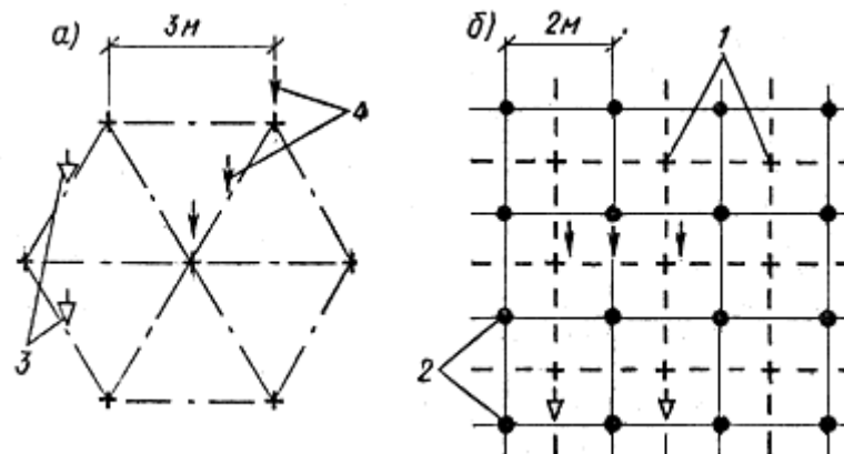
Рис.21. Схемы выполнения работ на участке опытного уплотнения песка
