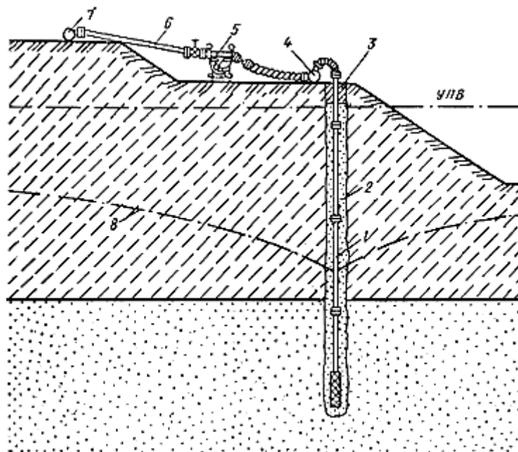
Рис.46. Схема понижения иглофильтрами в двухслойной среде
