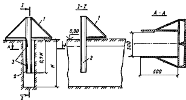
Рис.83. Кондуктор для монтажа стеновых панелей 1 - опорная рама; 2 - кондуктор; 3 - прижимная пружина
