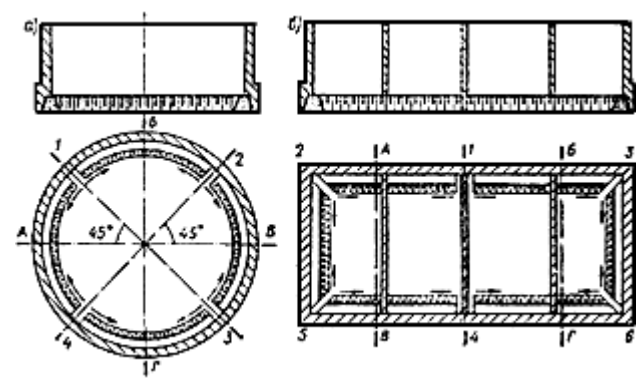
Рис.93. Схемы разработки опорных песчано-щебенистых призм при снятии опускного колодца или кессона с временного основания
