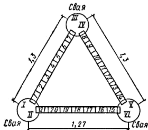
Рис.18. Схема отбора образцов грунта для определения плотности грунта 1-21 - места отбора образцов между грунтовыми сваями; I-VI - места отбора образцов в сваях
