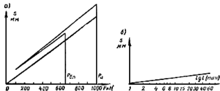
Рис.2. Приемочные испытания анкеров
