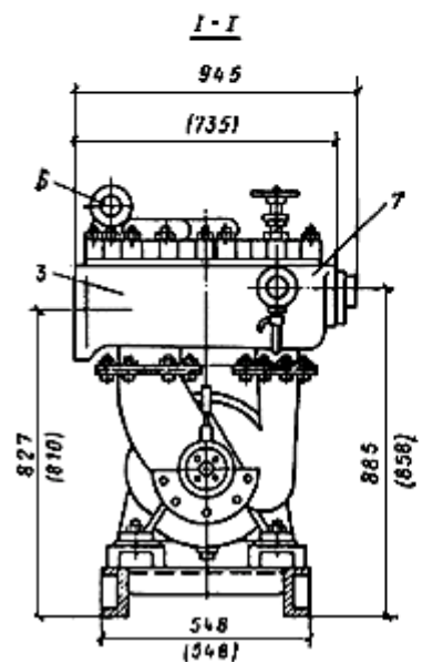
Рис.47. Насосная установка ЛИУ-6Б 1 - центробежный насос; 2 - вакуум-насос; 3 - колпак; 4 - электродвигатель; 5 - опорная рама; 6 - вакуумметр; 7 - манометр; 8 - фрикционная муфта
