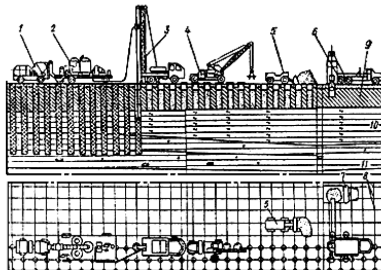
Рис.1. Укрепление основания буромесительным способом с использованием серийной буровой установки с работающим в непосредственной близости от нее растворонасосным узлом, смонтированным на передвижном шасси
