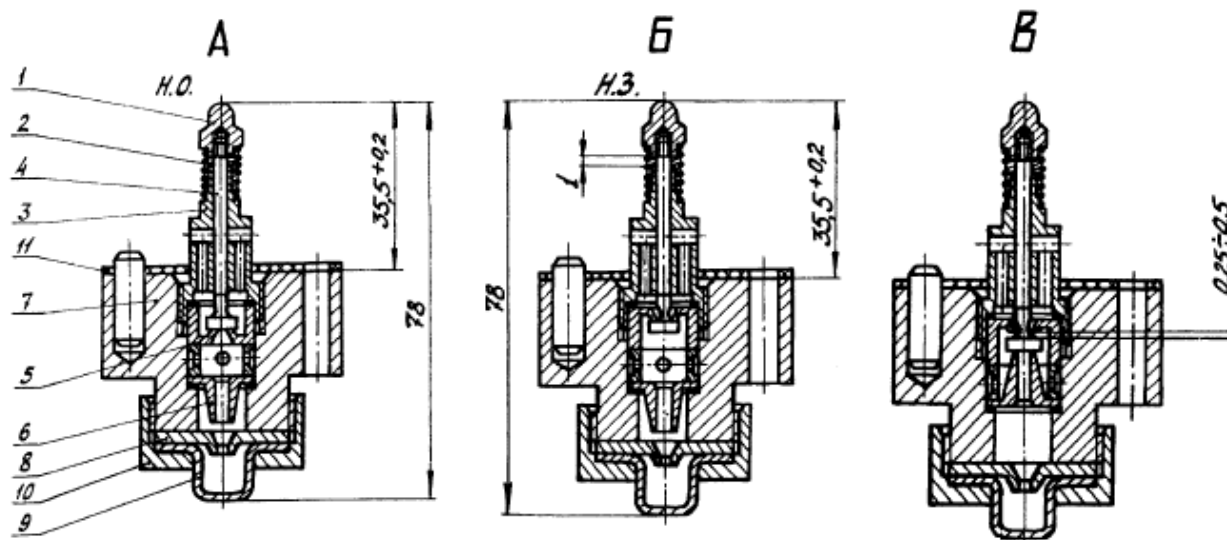
Рисунок АЖ.3.2 - Варианты сборки управляющего клапанка РД-3М
