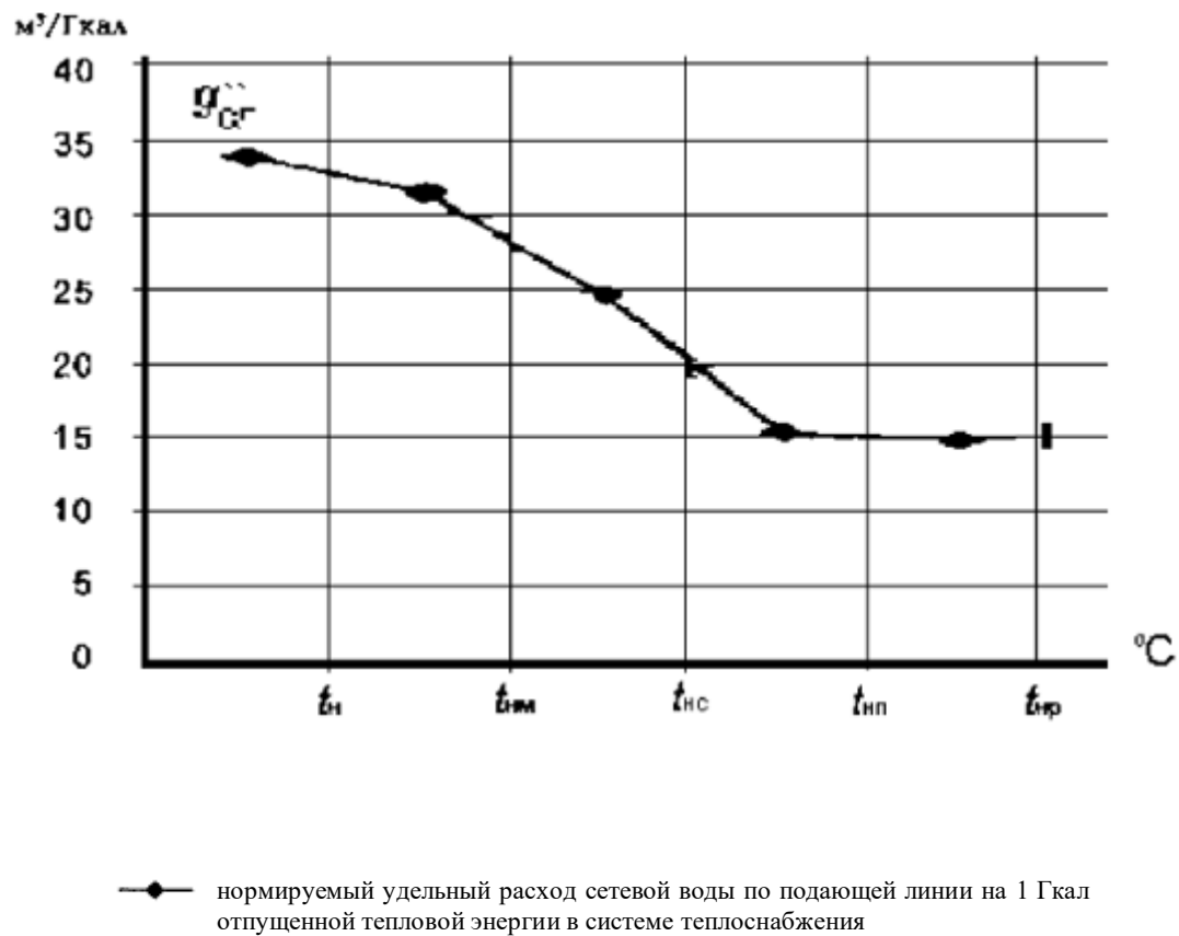
Рисунок АТ.Е.1 - График изменения нормируемого удельного расхода сетевой воды в подающем трубопроводе при характерных значениях температуры наружного воздуха
