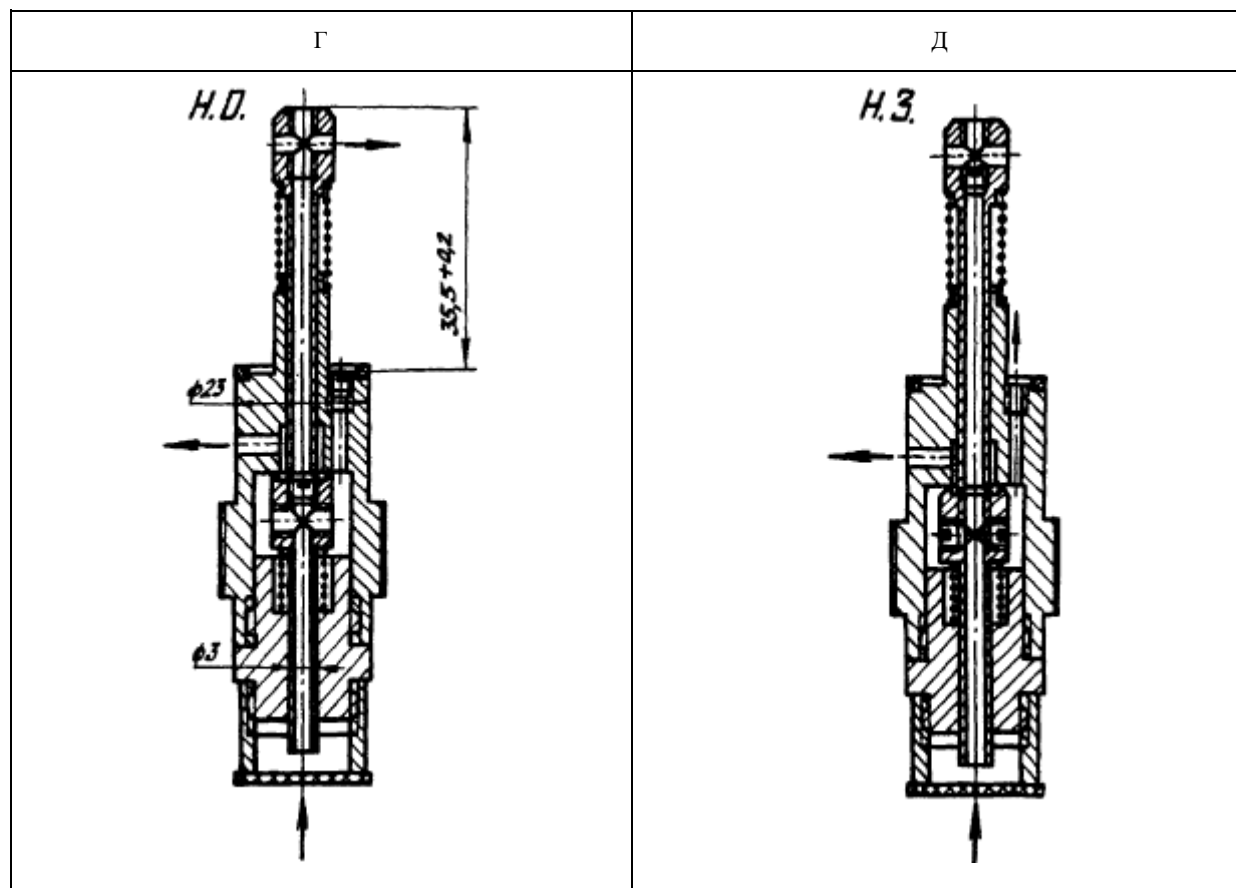
Рисунок АЖ.2.4 - Варианты сборки управляющего клапанка АЧ
