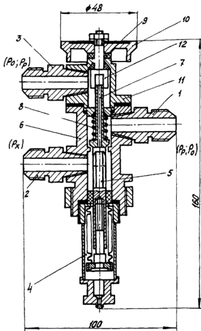
Рисунок АЖ.4.1 - Преобразователь температуры ПТ-1
