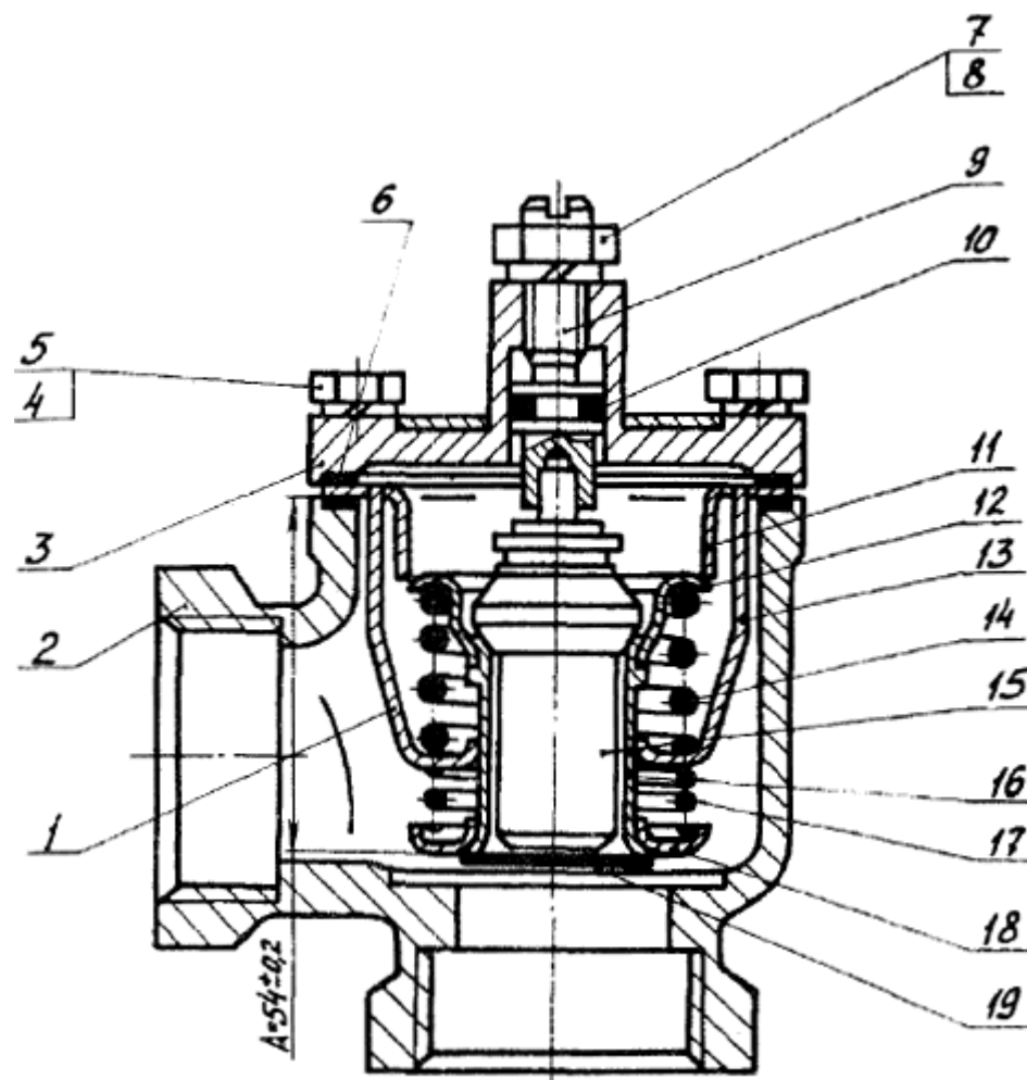
Рисунок АЖ.9.1 - Регулятор РТЦГВ
