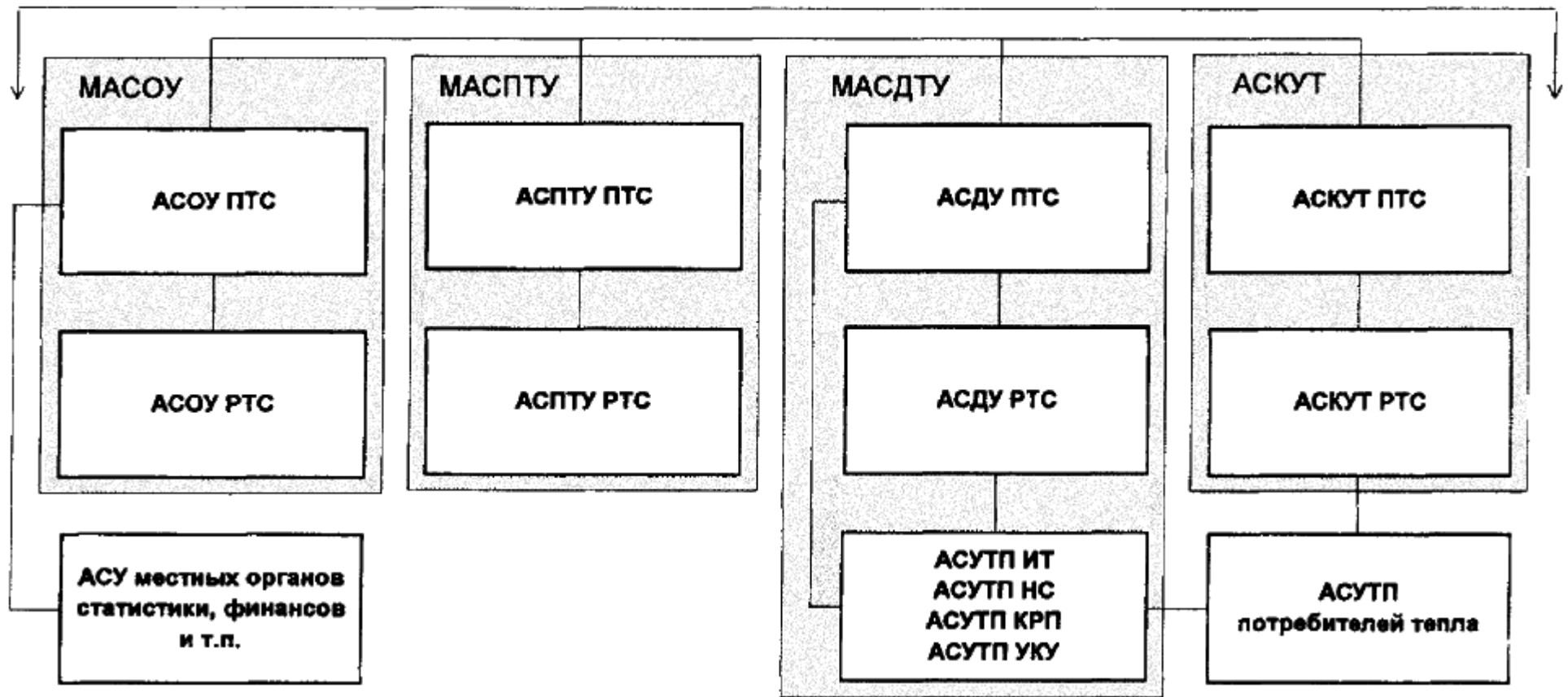
Рисунок БД.е.2.2 - Типовая функциональная структура ИАСУ "Теплосеть"
