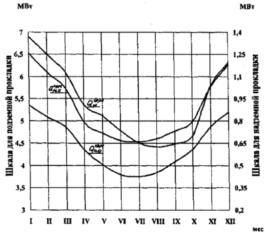
Рисунок АШ.Б.3 - Нормируемые часовые тепловые потери через теплоизоляционные конструкции при среднемесячных условиях
