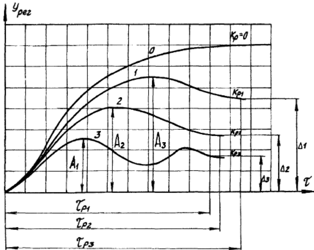
Рисунок АЛ.1 - Переходные процессы в замкнутой системе с пропорциональным регулятором при изменении коэффициента усиления регулятора
