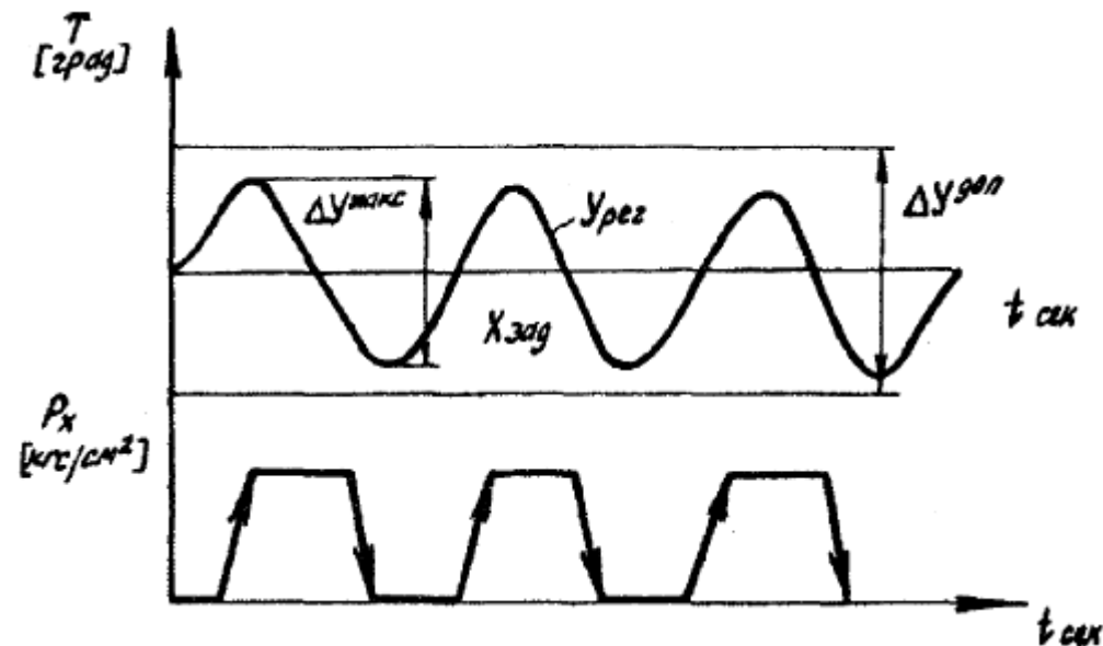
Рисунок АЖ.5 - График процесса регулирования температуры ГВС регулятором ПТ-1
