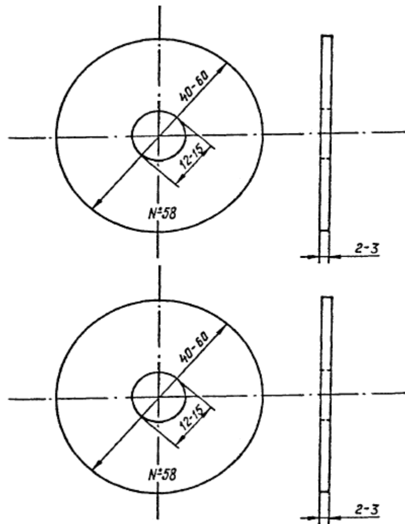
Рисунок У.1 - Индикатор внутренней коррозии
