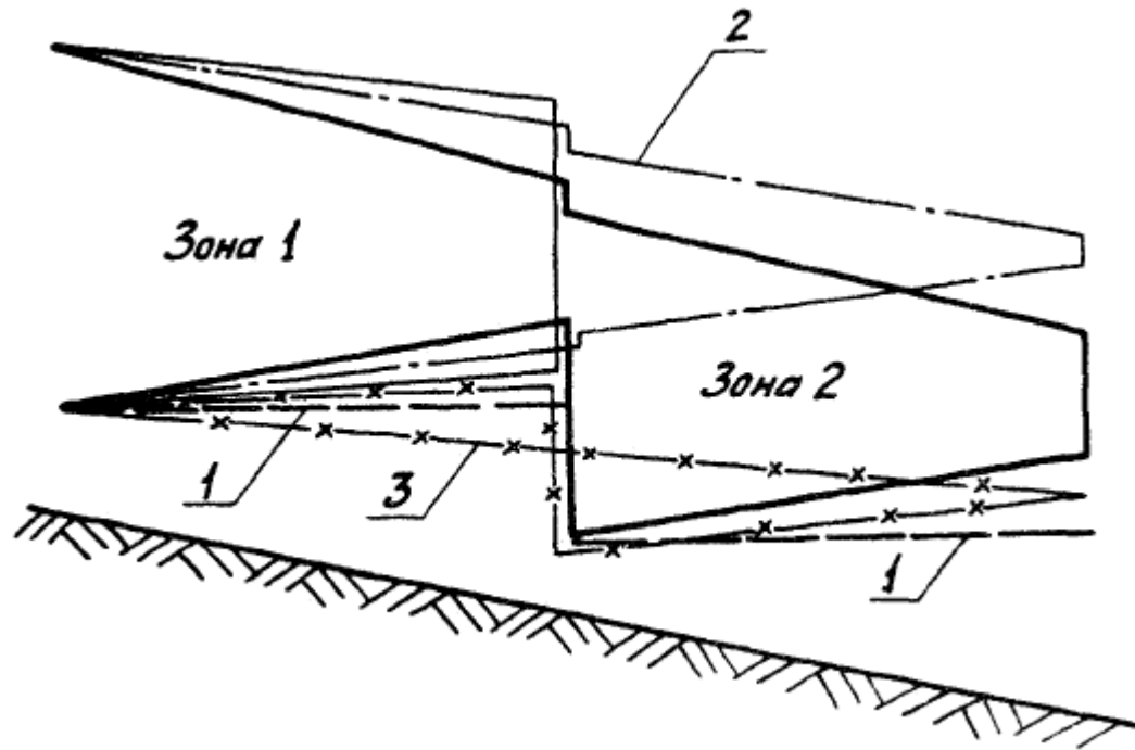
Рисунок АЖ.21 - Пьезометрический график тепловой сети
