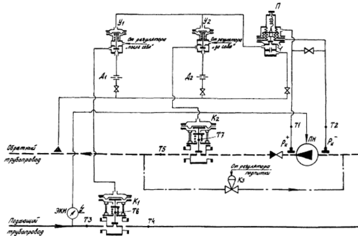
Рисунок АЛ.8 - Схема автоматического управления устройством рассечки
