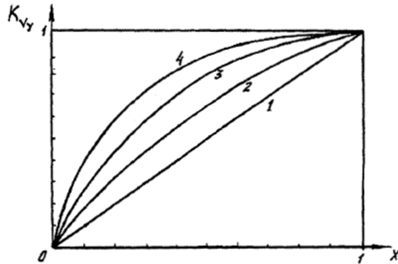
Рисунок АЖ.7 - График расходной характеристики РО
