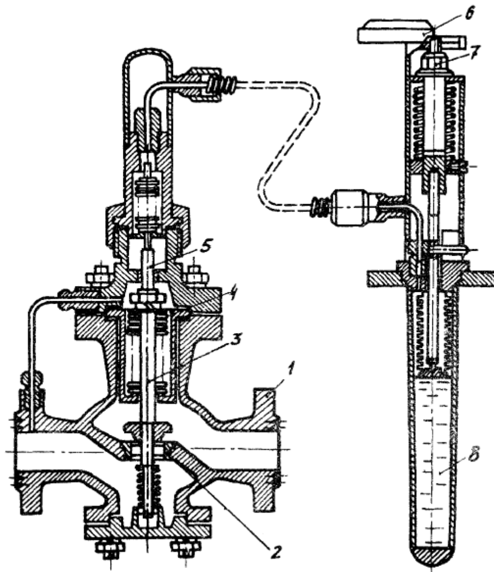
Рисунок АЖ.8.1 - Регулятор температуры прямого действия РТ-ДО (ДЗ)
