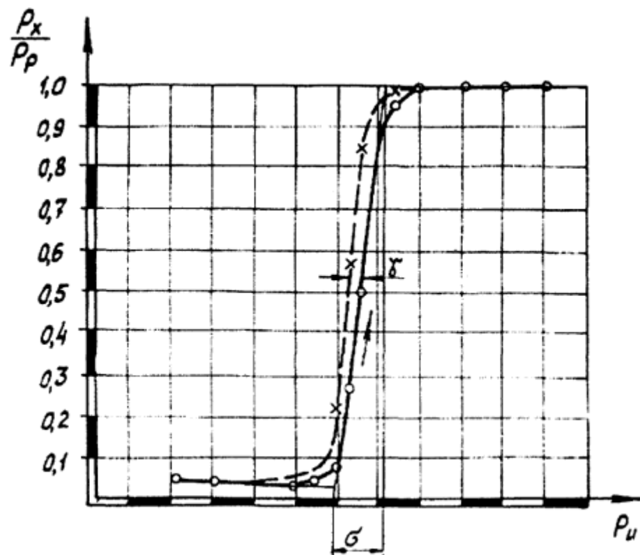
Рисунок АЖ.9 - Статическая характеристика регулирующего прибора РД-3А
