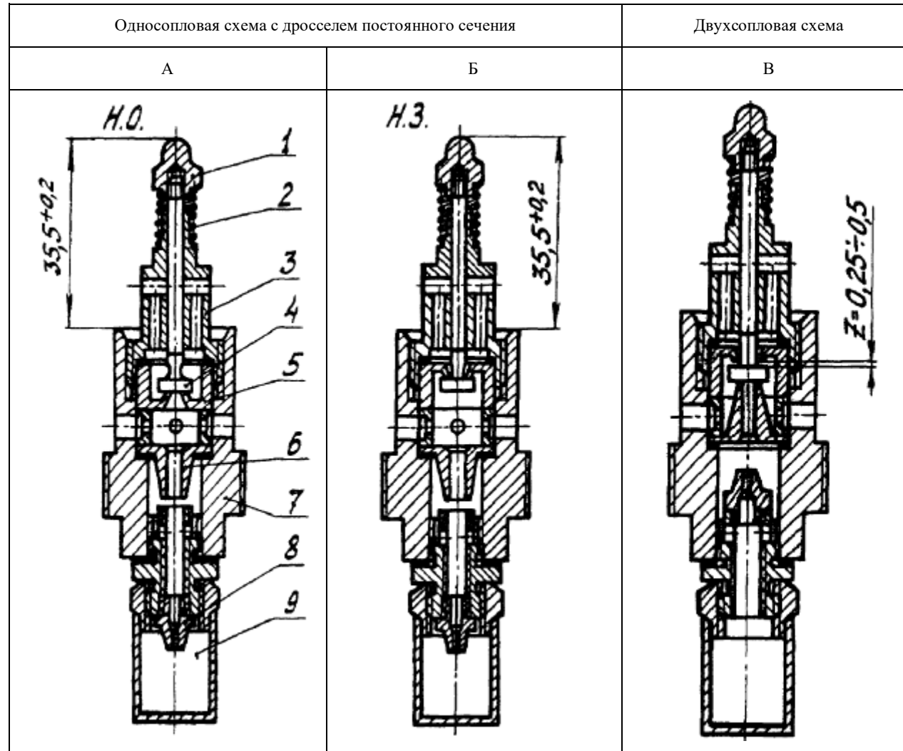
Рисунок АЖ.2.3 - Варианты сборки управляющего клапанка
