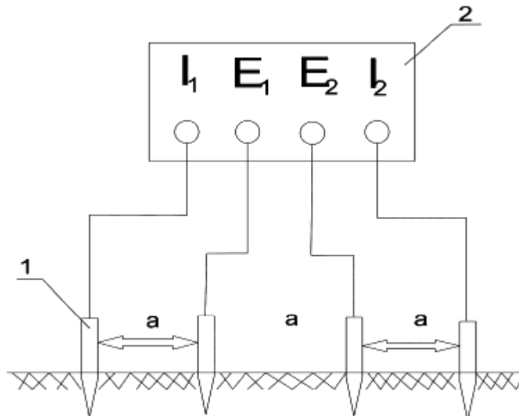
1 - стальные электроды; 2 - измерительный прибор
