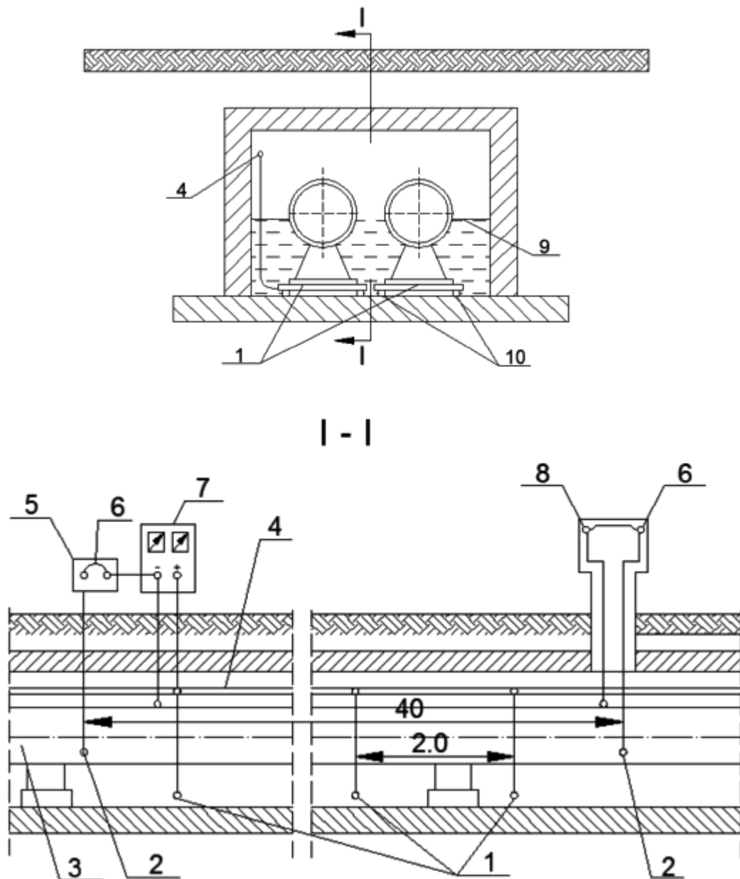
1 - электроды АЗ стержневого типа; 2 - вспомогательные электроды; 3 - трубопровод; 4 - распределительный кабель; 5 - КИП у станции катодной защиты; 6 - электроперемычка; 7 - станция катодной защиты (преобразователь); 8 - КИП; 9 - уровень затопления канала; 10 - диэлектрические опоры
