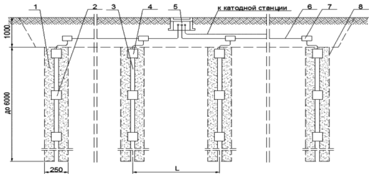
Рисунок В.7 - Поверхностное АЗ с горизонтальным размещением железокремнистых электродов
