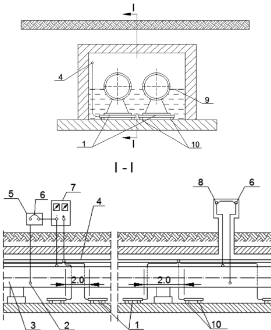
1 - электроды АЗ стержневого типа; 2 - вспомогательный электрод; 3 - трубопровод; 4 - распределительный кабель; 5 - КИП у станции катодной защиты; 6 - электроперемычка; 7 - станция катодной защиты (преобразователь); 8 - КИП; 9 - уровень затопления канала; 10 - диэлектрические опоры
